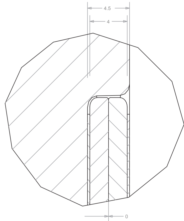
DETTAGLIO A SCALA 5:1
