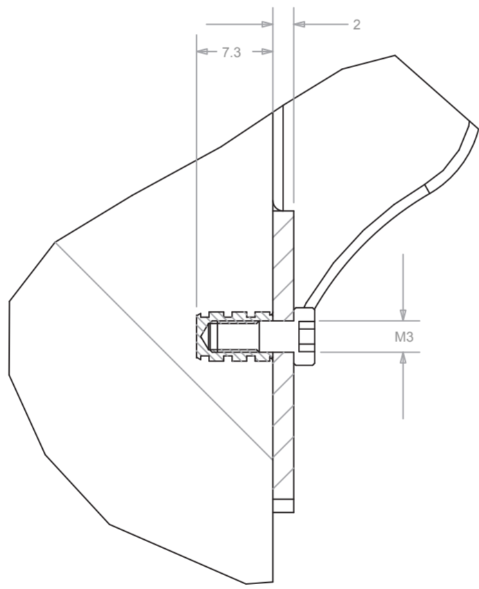
DETTAGLIO B SCALA 2:1
