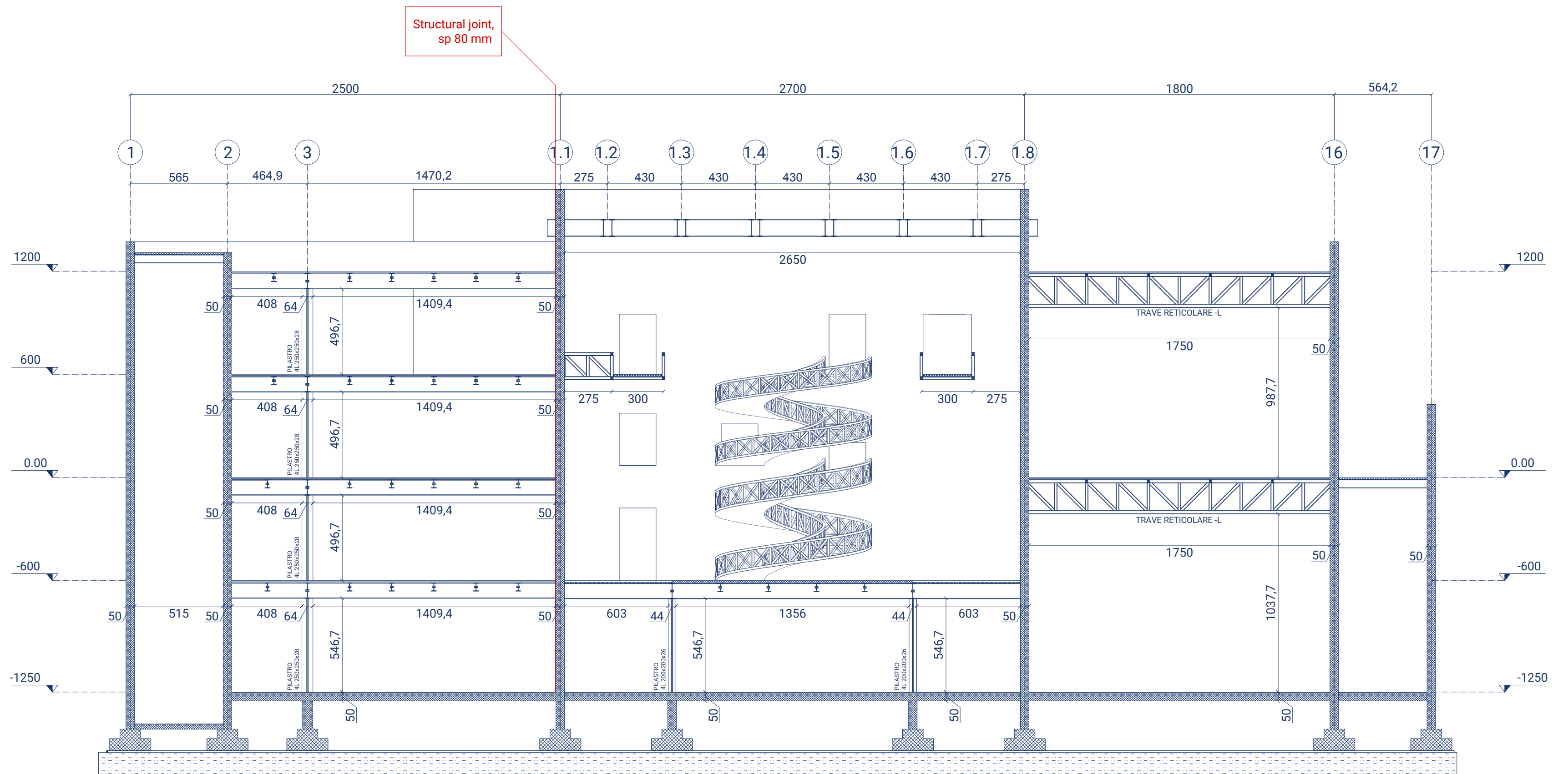
Sezione trasversale strutturale
