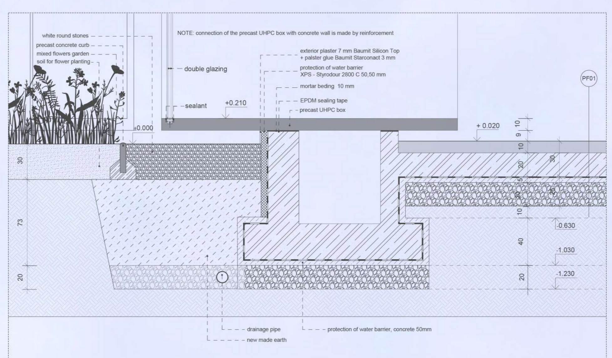
D2 1/20
