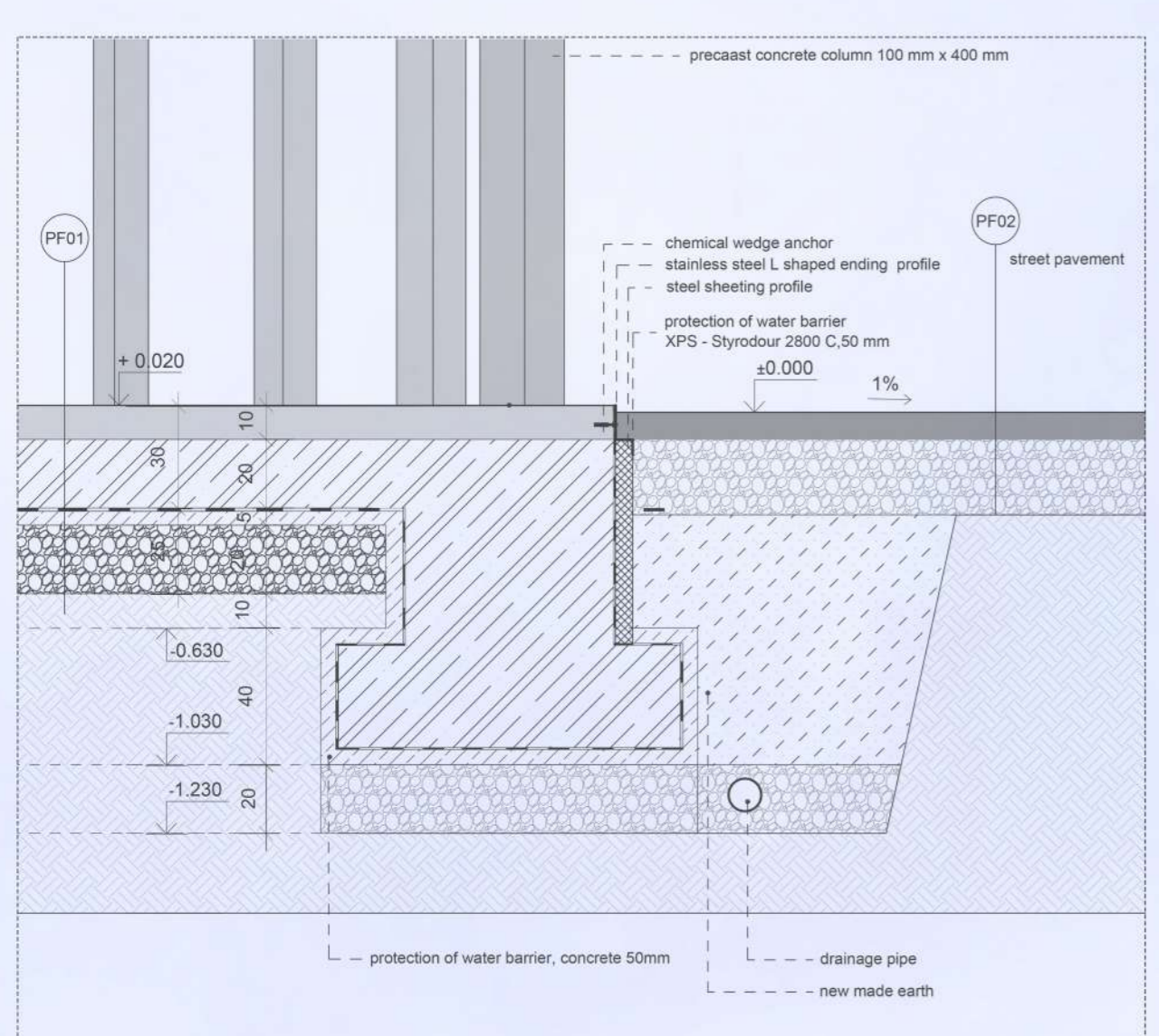
D1 1/20
