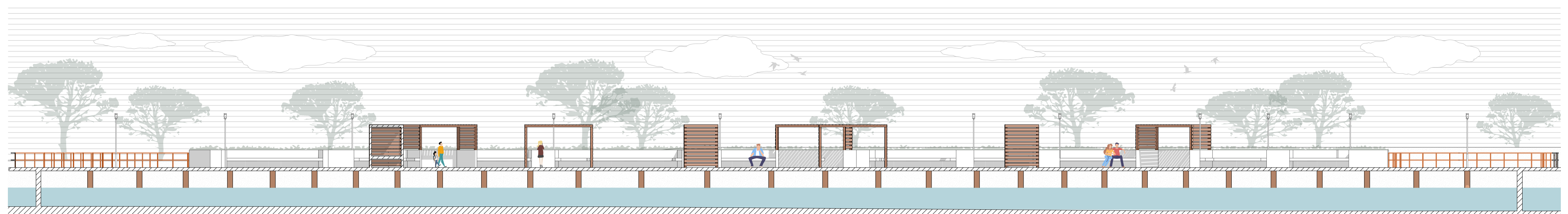
SEZIONE DD' _ 1:200
