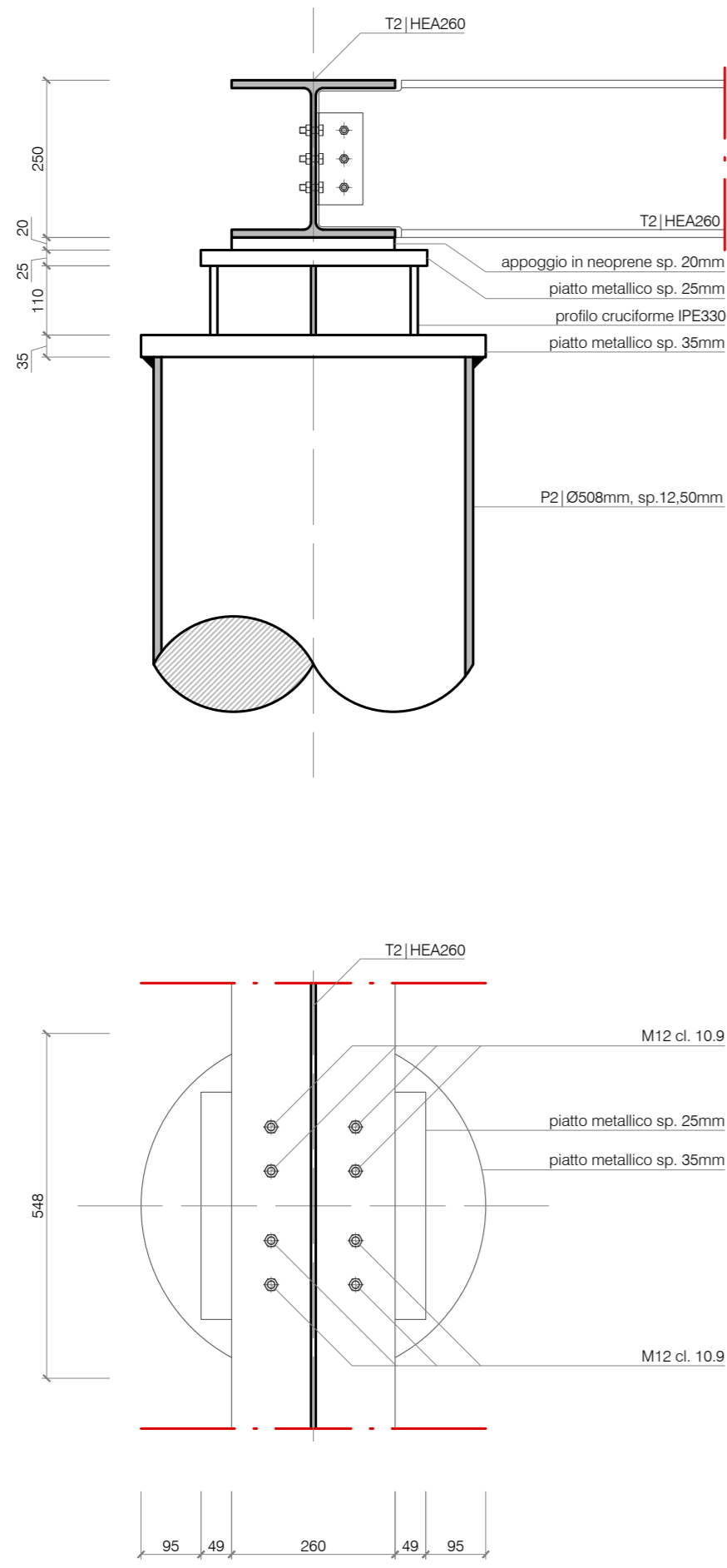
DETTAGLIO STRUTTURA IN ACCIAIO Sistema di appoggio trave custom su pilastro cruciforme Scala 1:10
