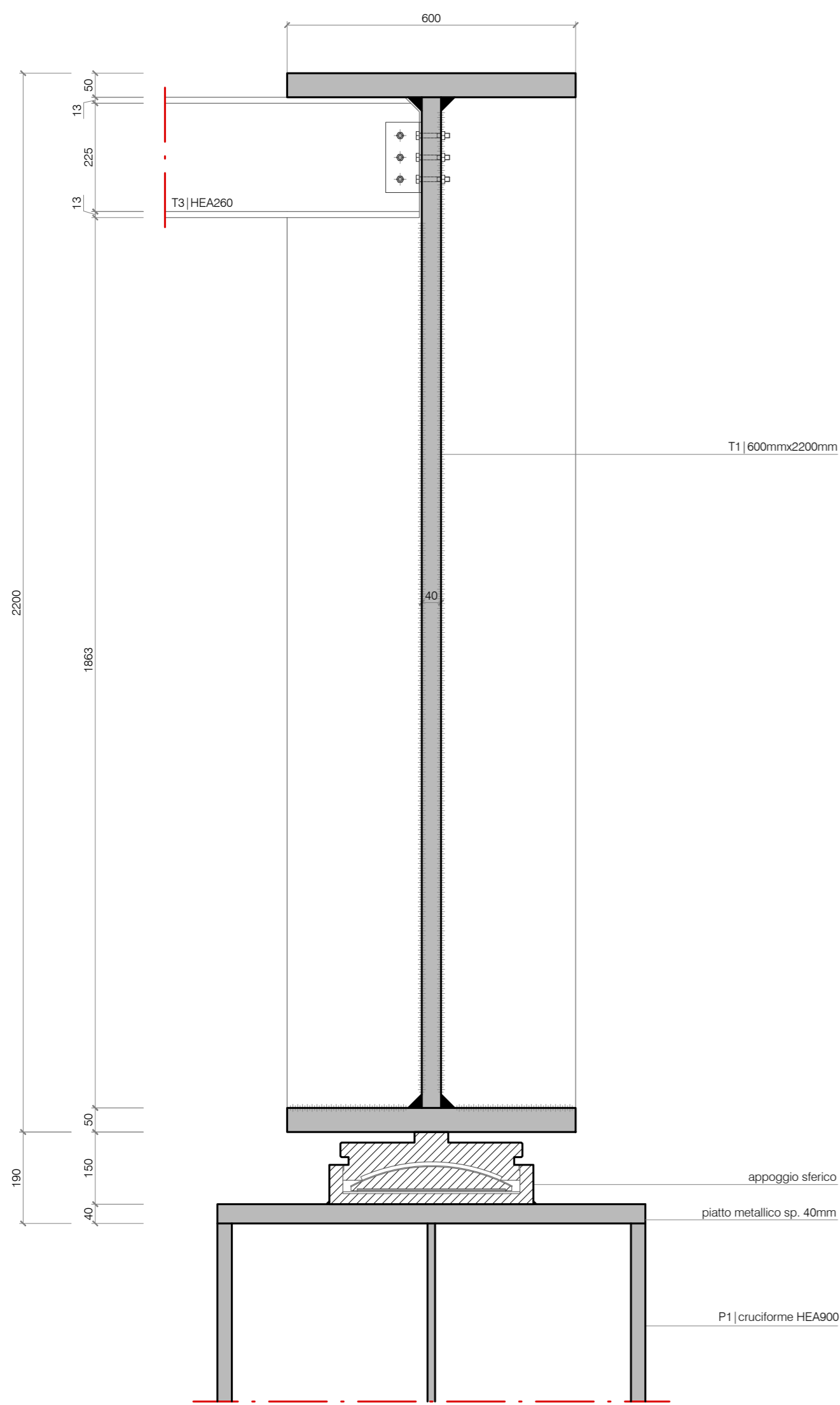
DETTAGLIO STRUTTURA IN ACCIAIO Sistema di appoggio trave custom su pilastro cruciforme Scala 1:10
