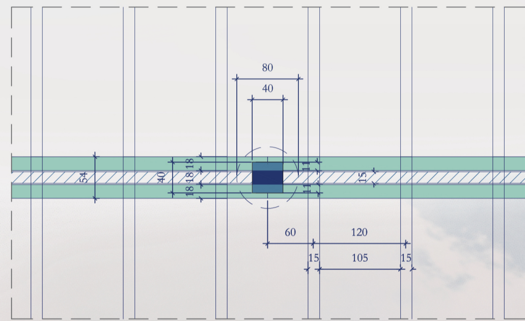
Nodo pilastro travi 1:50
