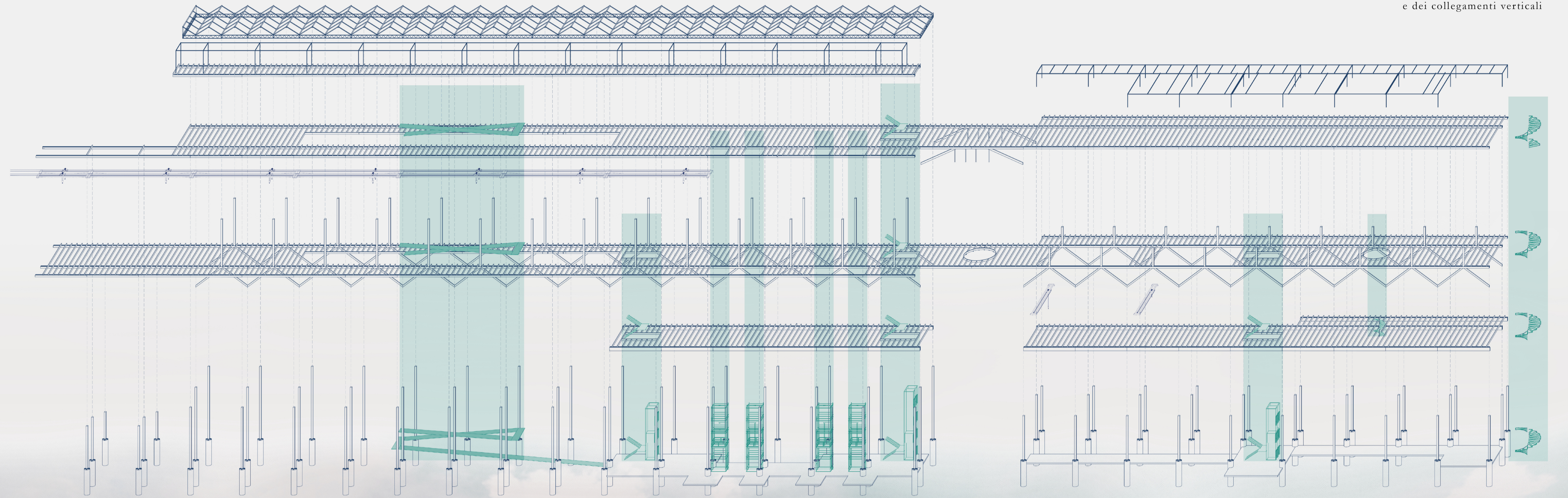
Esploso assometrico delle componenti strutturali lignee e dei collegamenti verticali
