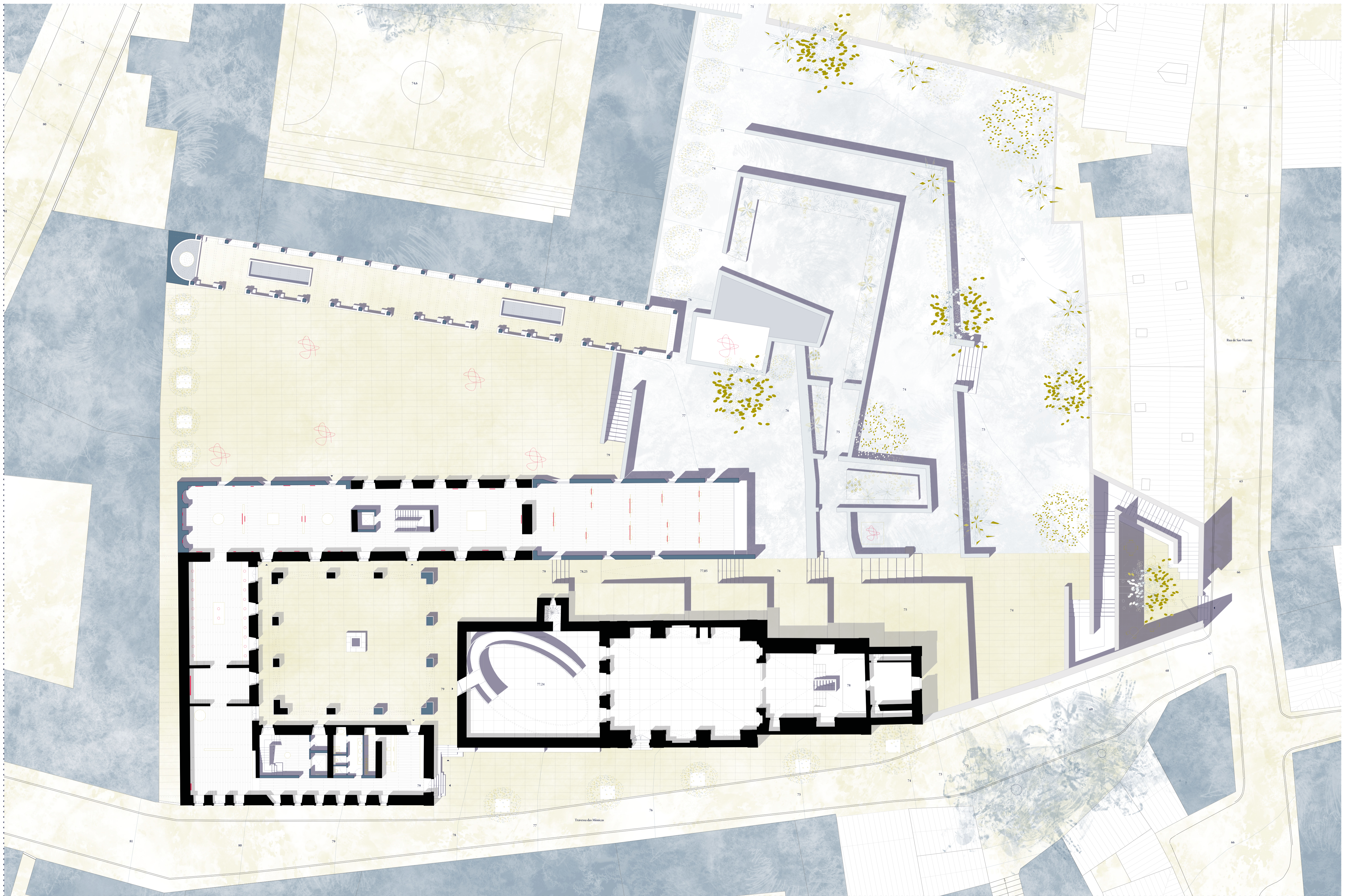
Pianta piano terra 1:200 Alice Serafini, Giulia De Matteis
