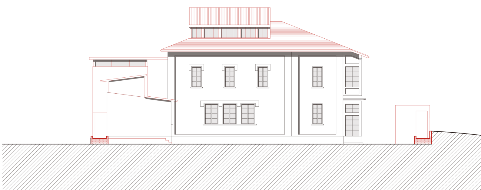
FACADE A-A 1:200
