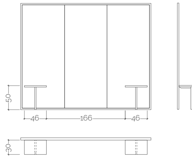
► Frame scala 1:50
