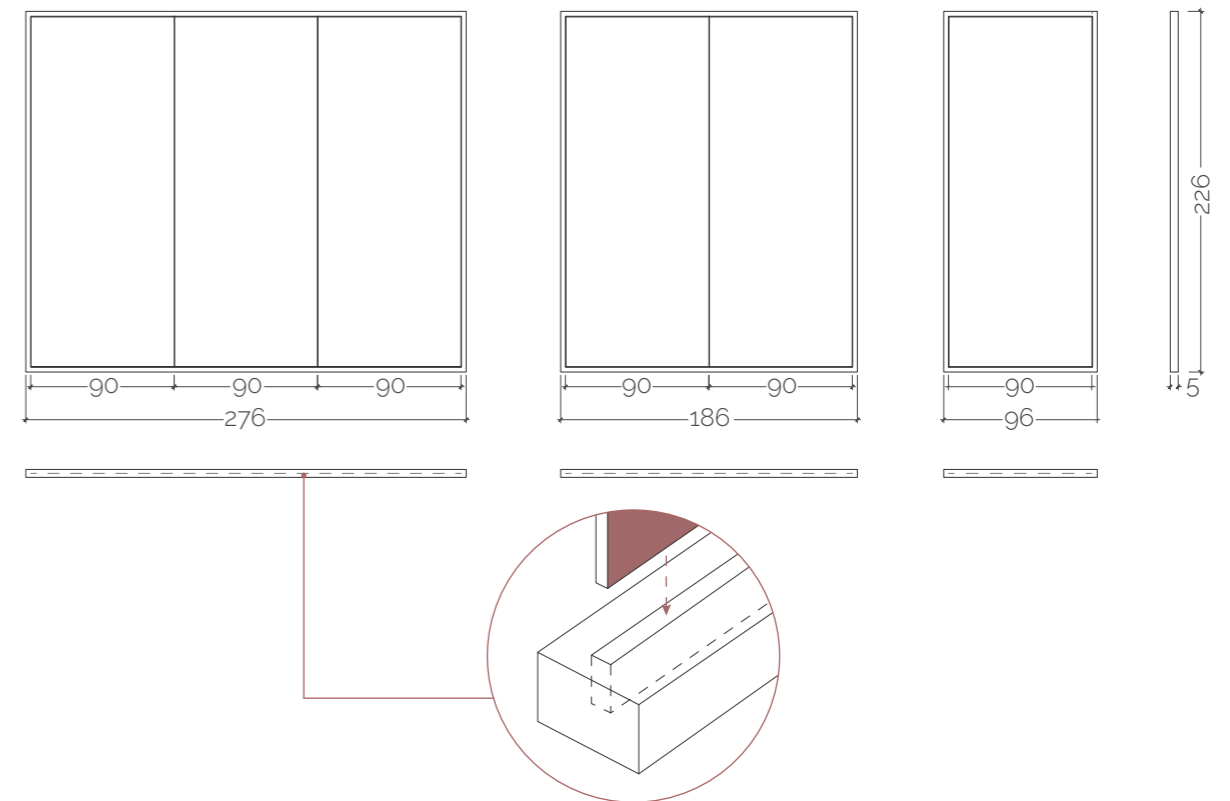
Dettaglio frame in scala 1:50
