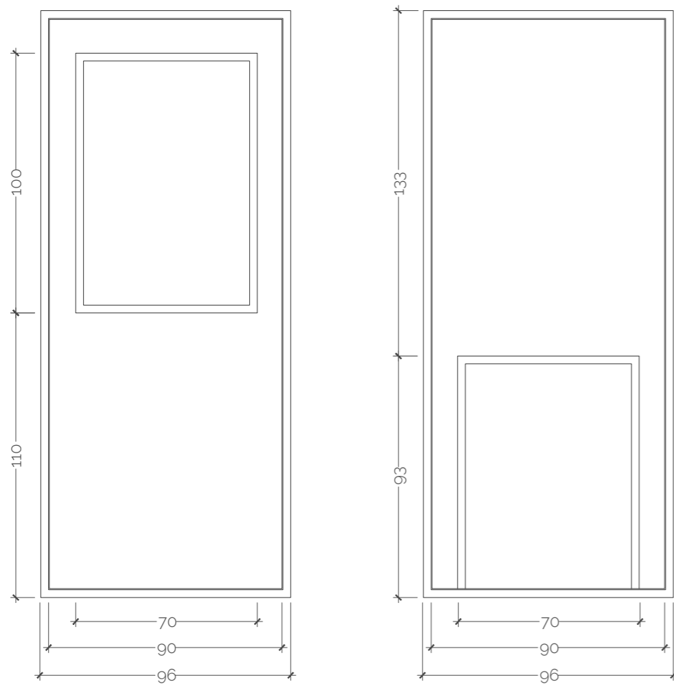
► Frame scala 1:20
