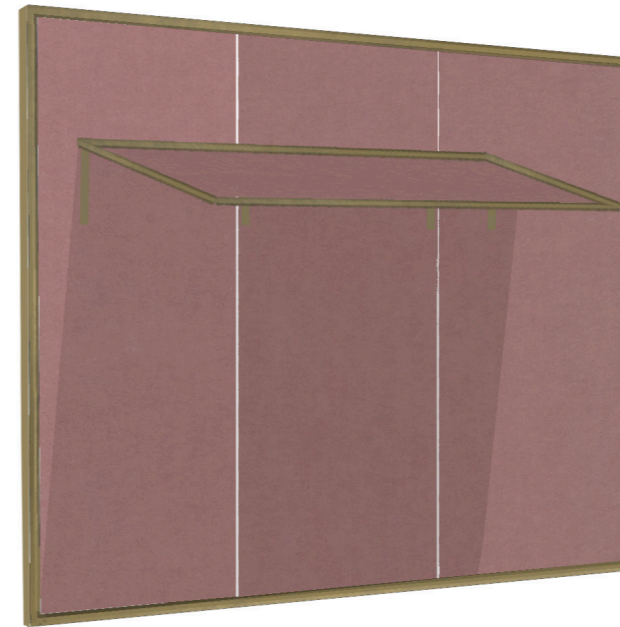
▶ B: Frame camera: copertura lunga 90 cm, inclinazione 60°
