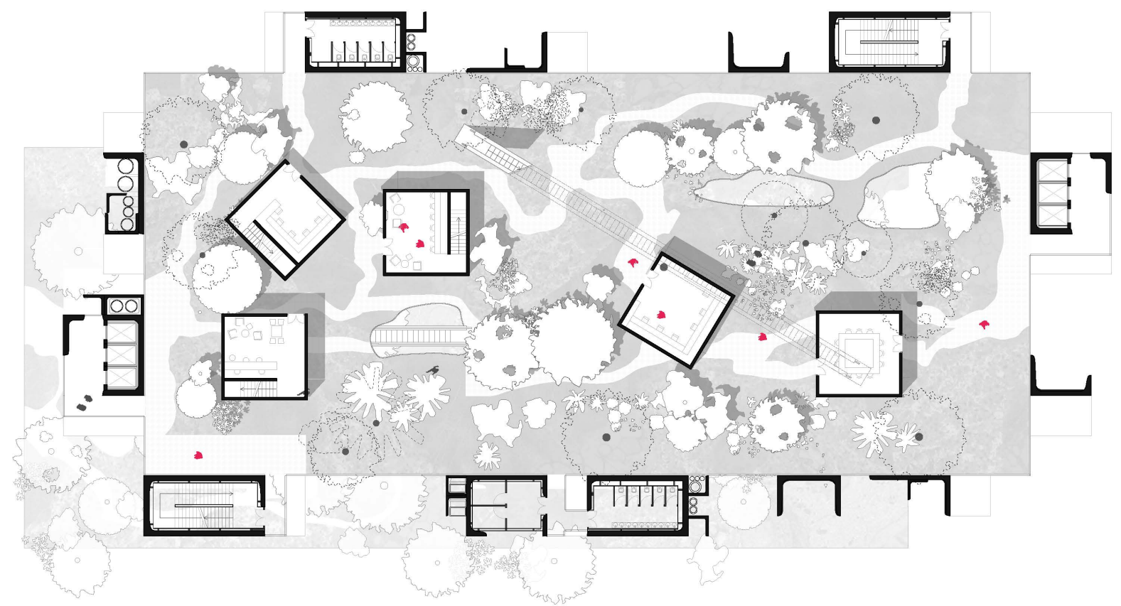
PIANTA LIVELLO 3 piano tipo
