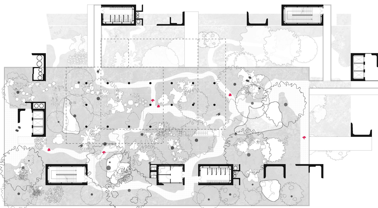
PIANTA LIVELLO 5
