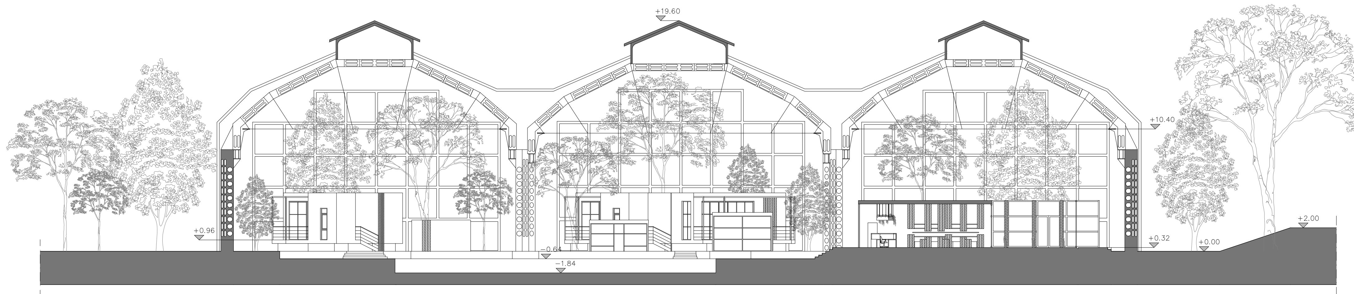
Sezione A-A'
