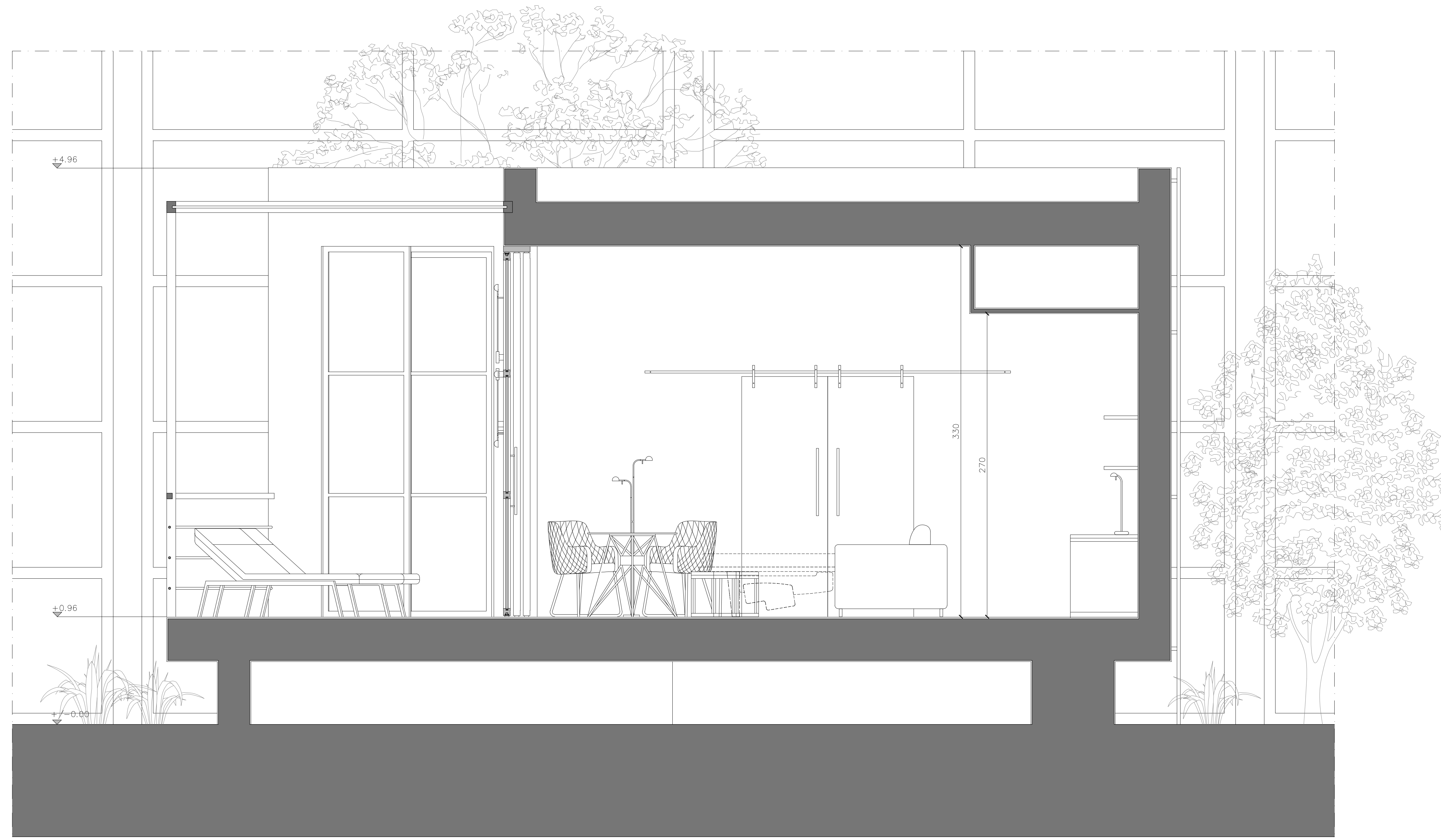
Sezione A-A'
