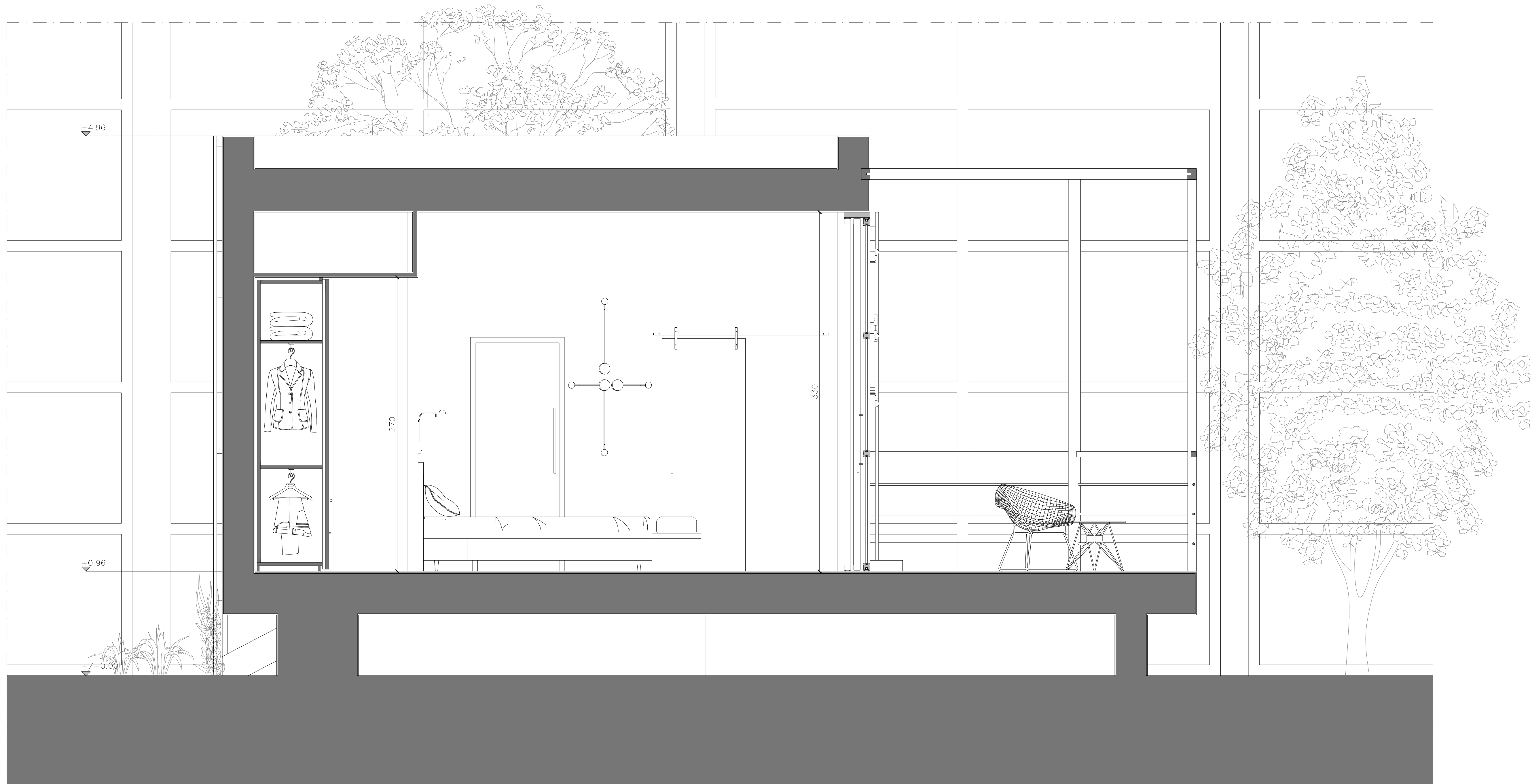
Sezione A-A'
