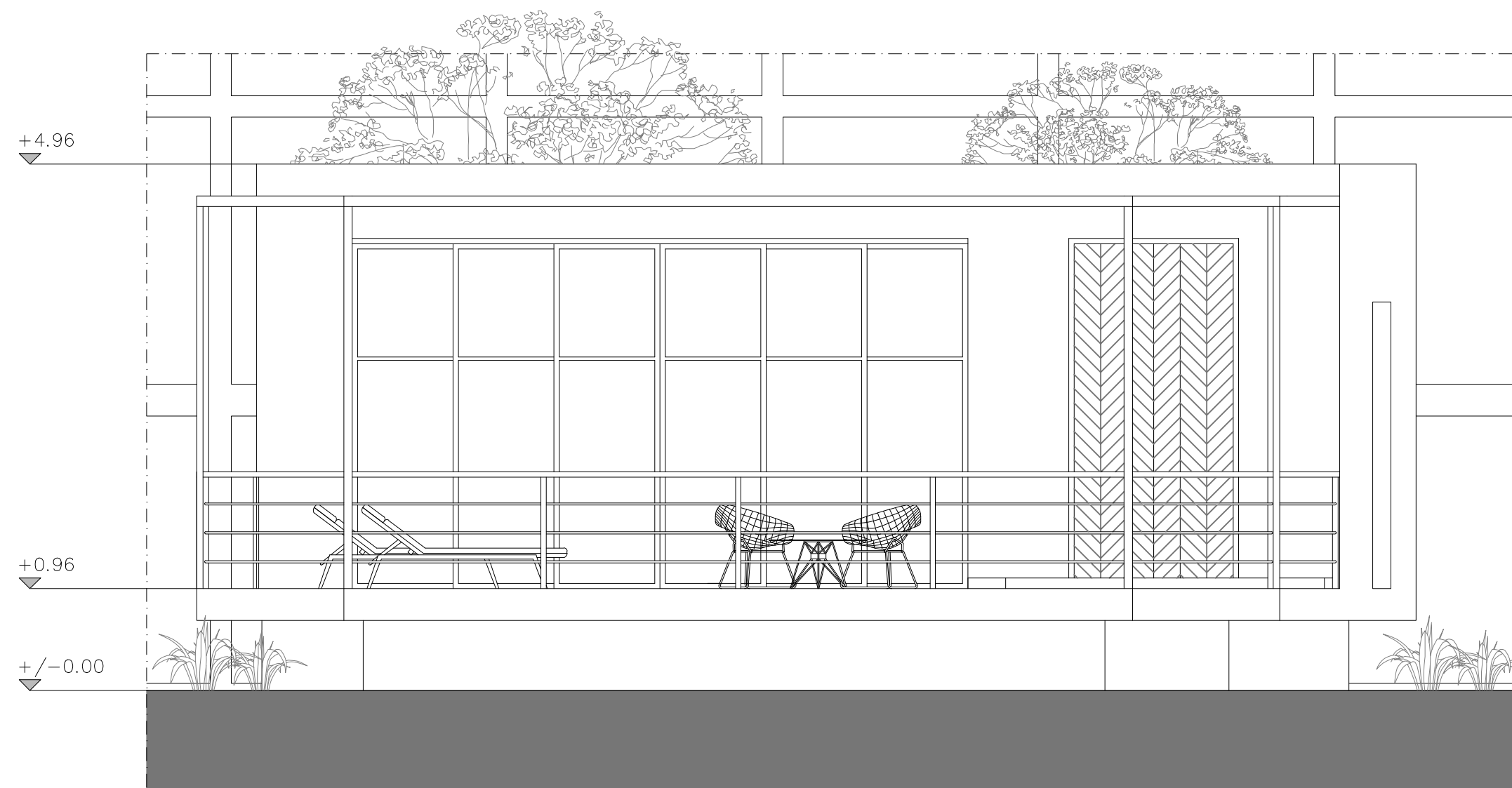
Prospetto terrazzo
