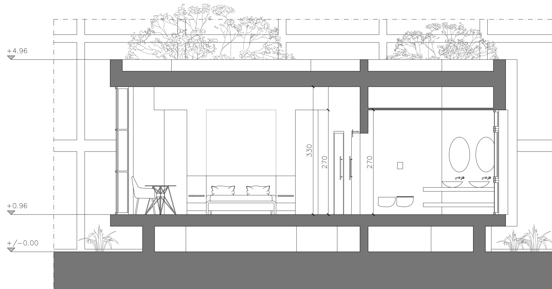
Sezione B-B'
