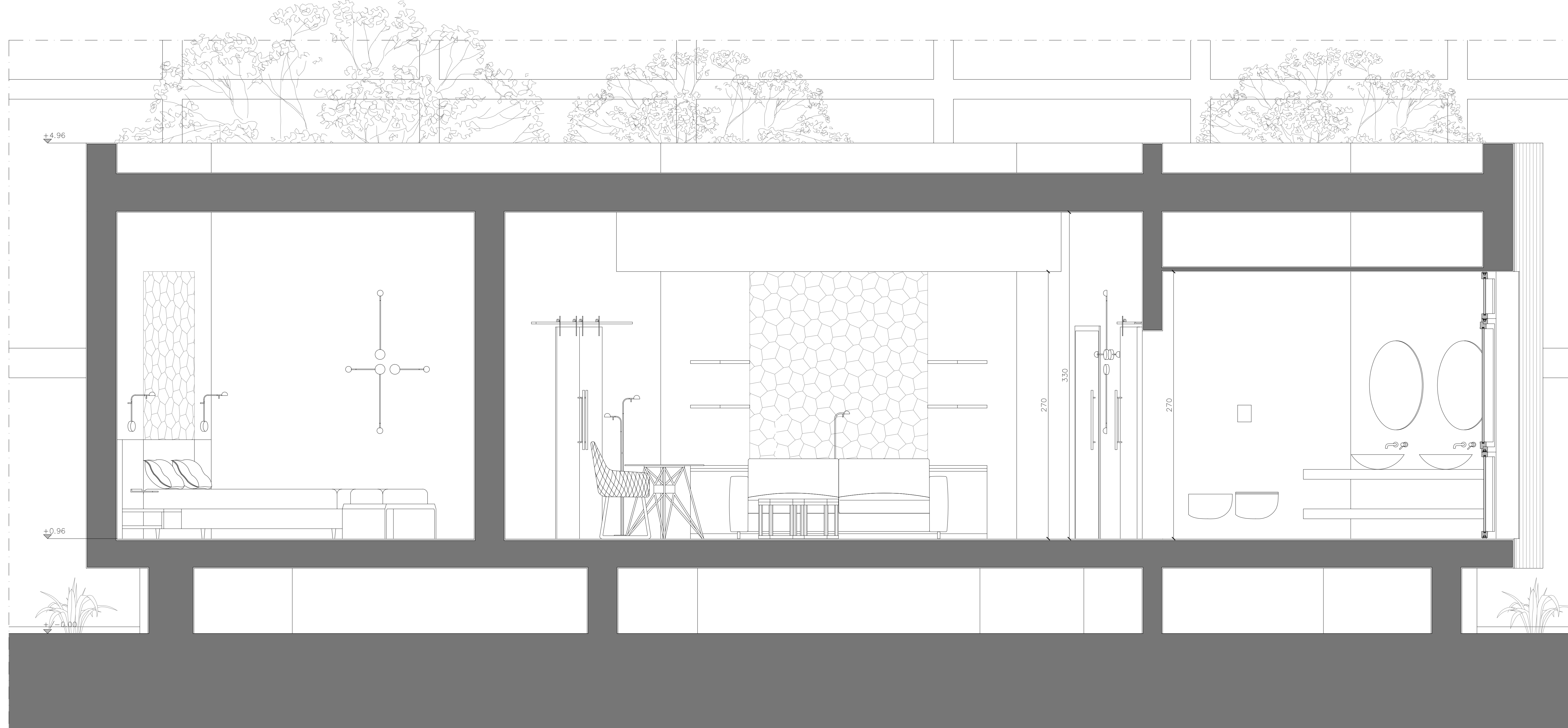
Sezione B-B'
