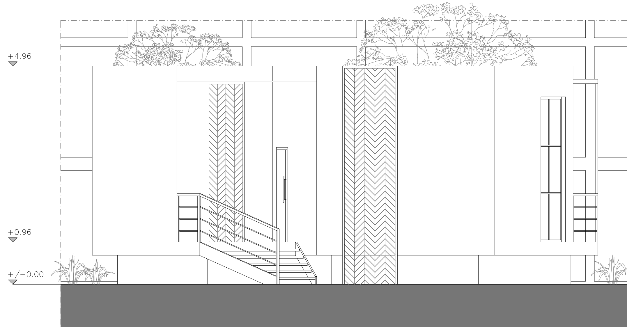
Prospetto ingresso
