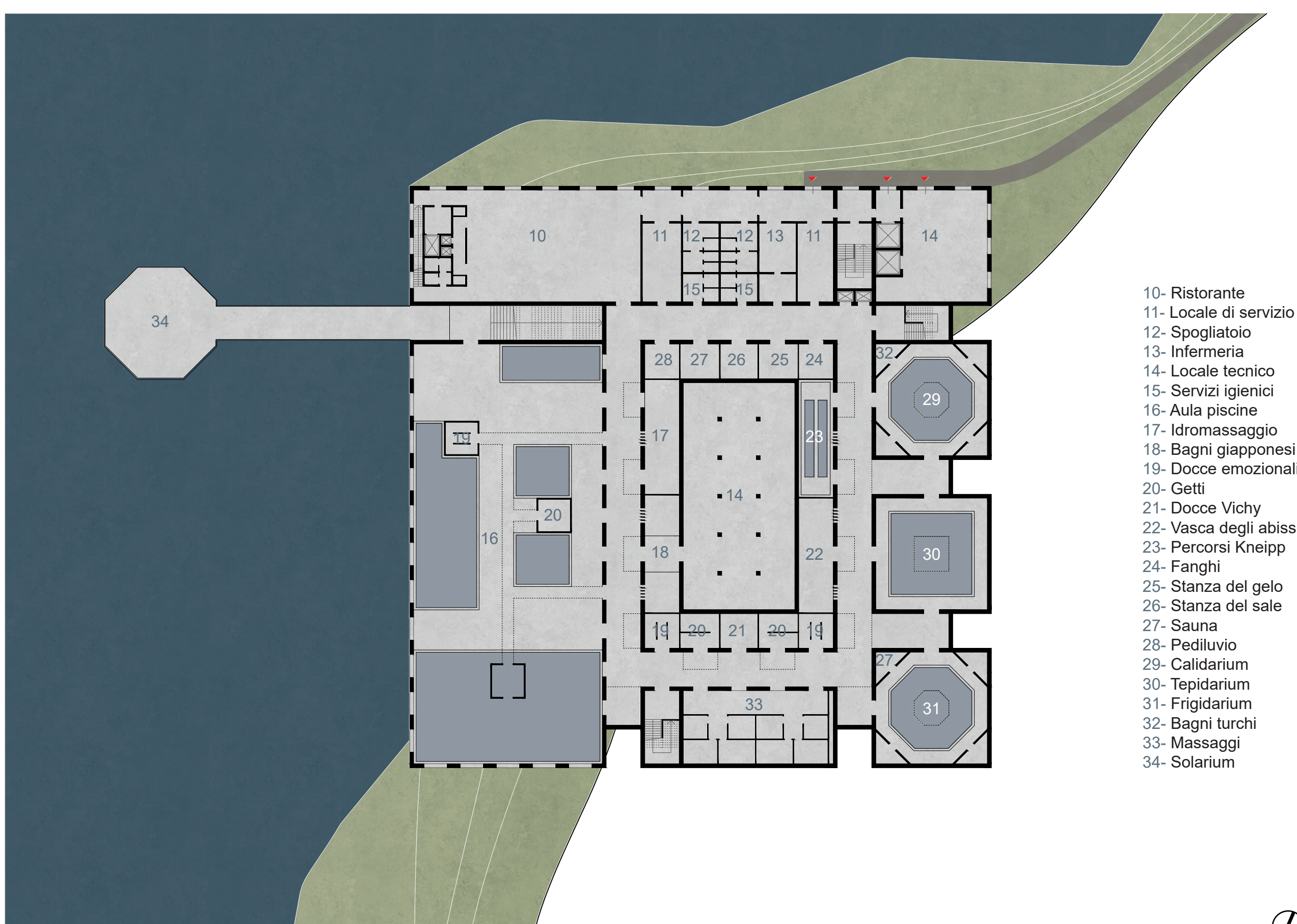
PIANTA LIVELLO -2
