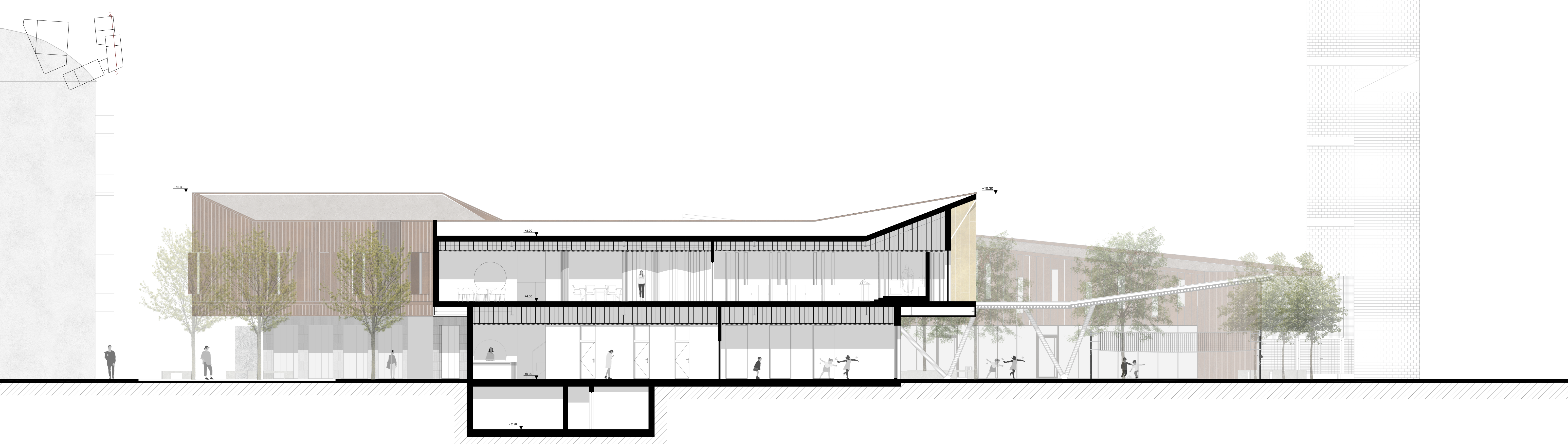
SEZIONE LONGITUDINALE E-E'
