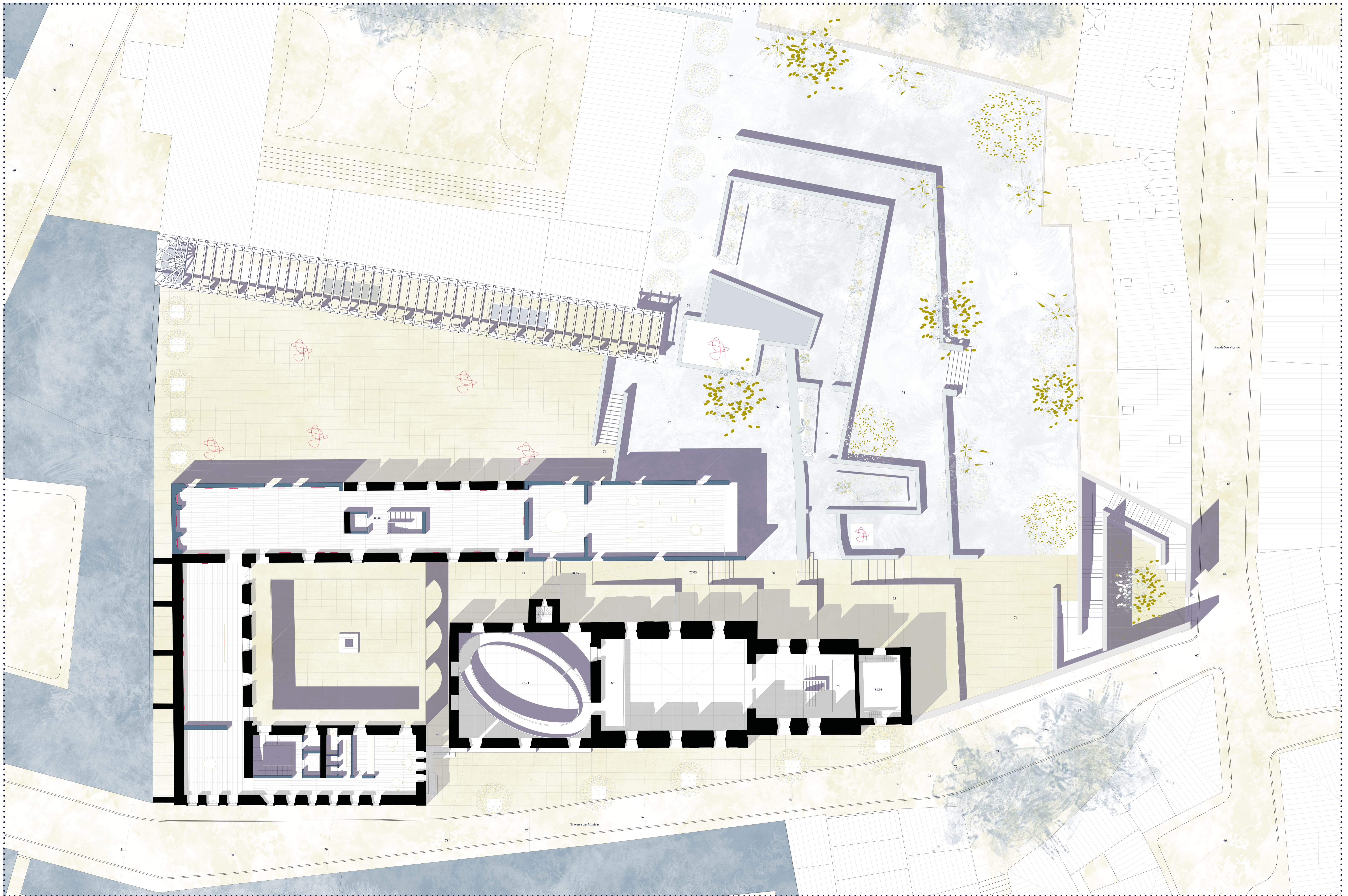
Pianta piano primo 1:200
