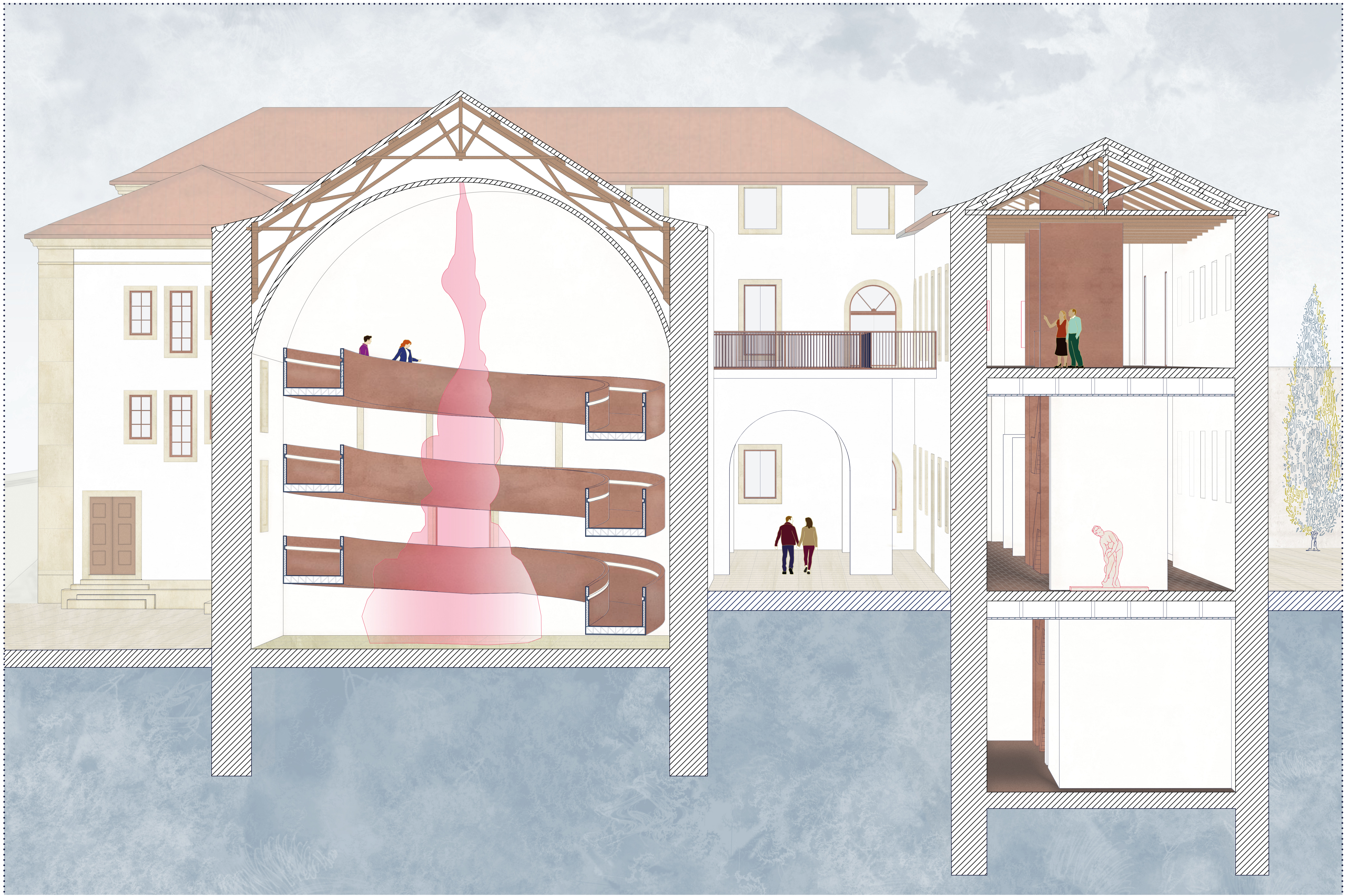
Sezioni 1:50 di dettaglio - Chiesa e Museo Alice Serafini, Giulia De Matteis
