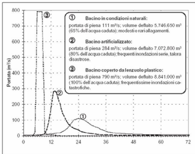
Figura 12: onda di piena per differenti condizioni di permeabilità del suolo
