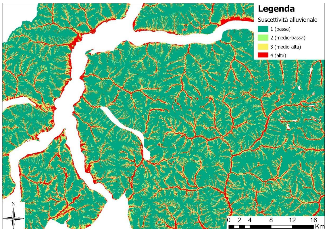
Figura 40: suscettività alluvionale in una porzione di territorio della “montagna”
