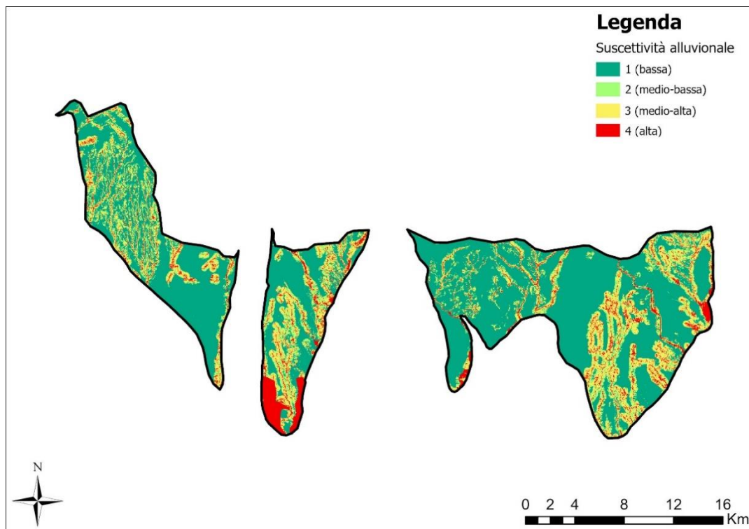
Figura 46: suscettività alluvionale in “collina tabulare”
