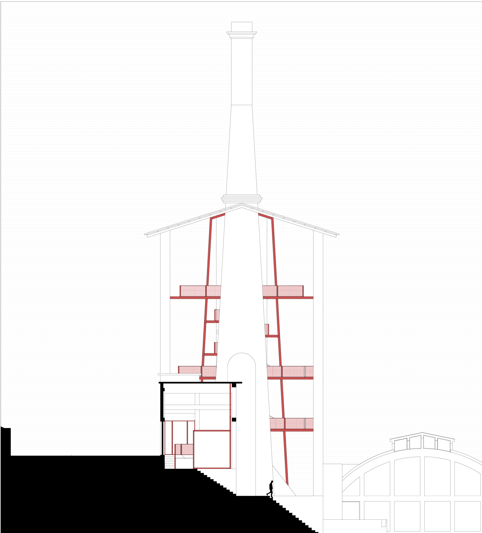
Sezione B-B'
