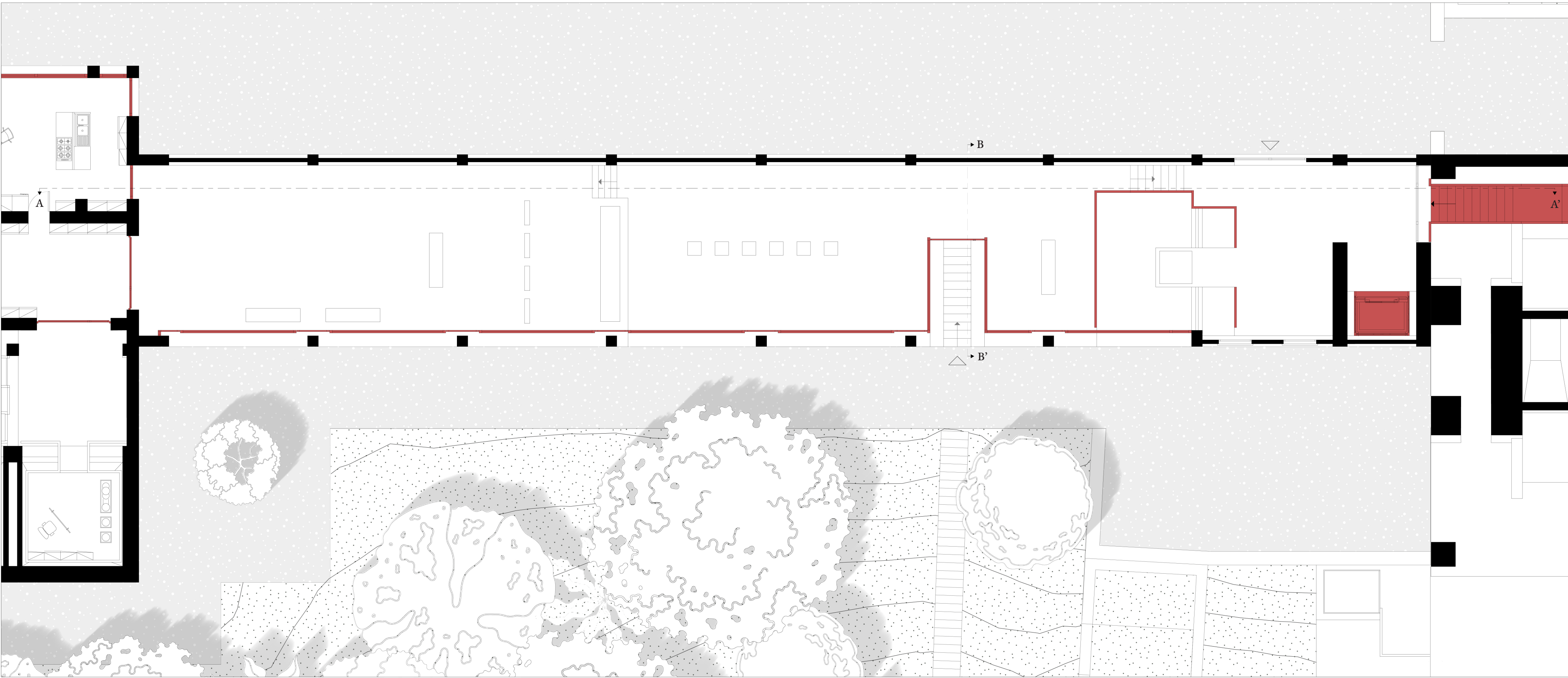
Pianta Piano Terra 1:100
