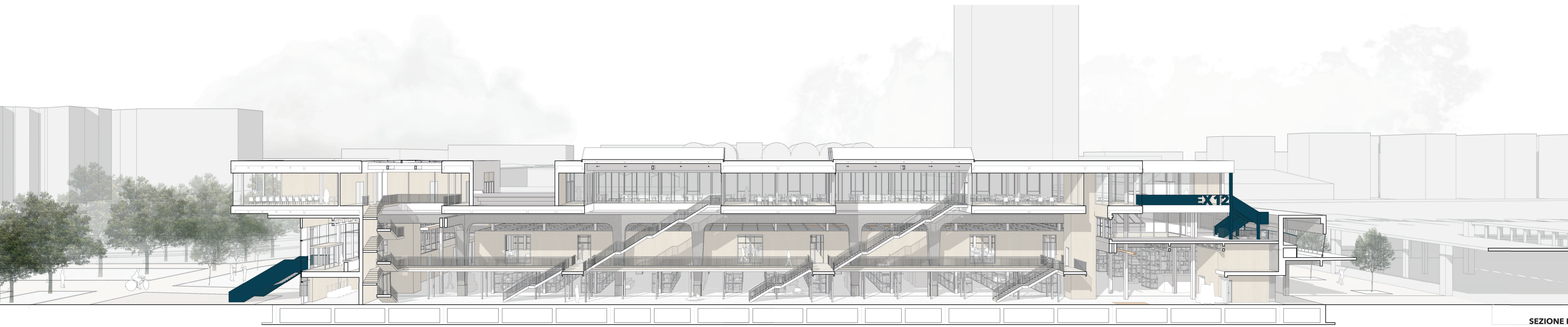
SEZIONE HH'
