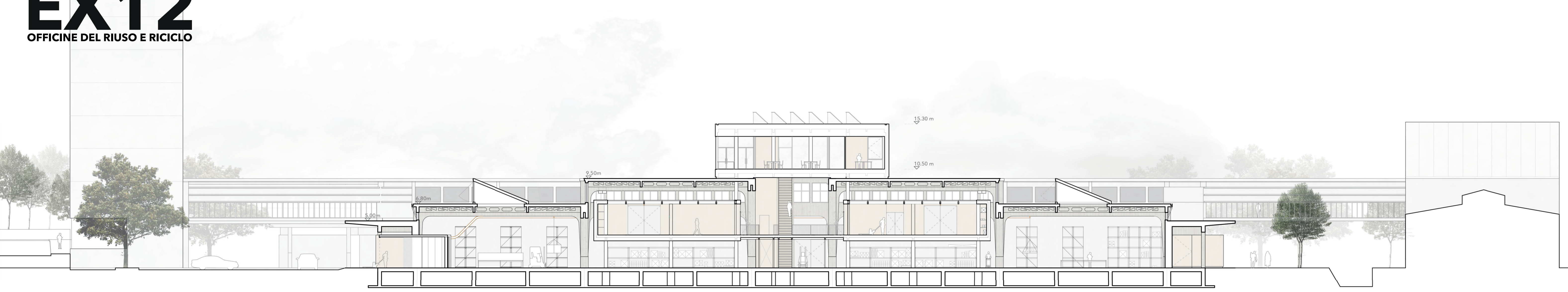
SEZIONE GG'
