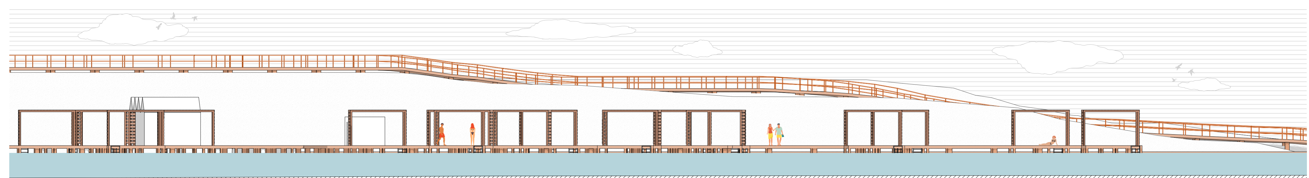
SEZIONE DD' _ 1:200
