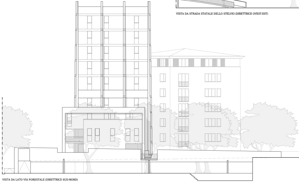
VISTA DA LATO VIA FORESTALE (DIRETTRICE SUD-NORD)
