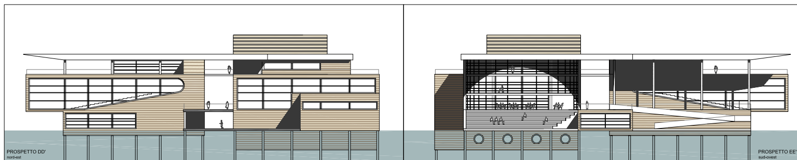
PROSPETTO DD' _ nord-est
