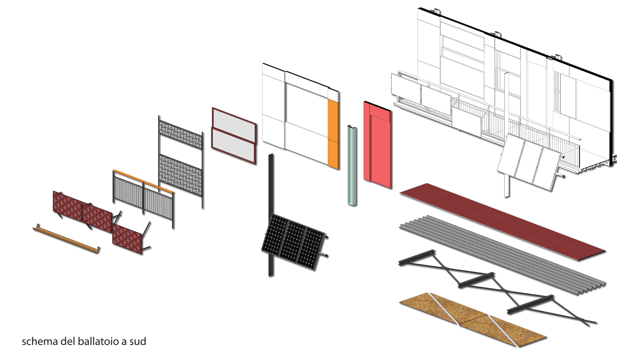
schema del ballatoio a sud
