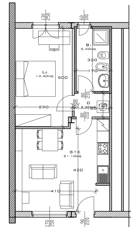
piante delle tipologie abitative - scala 1:100
