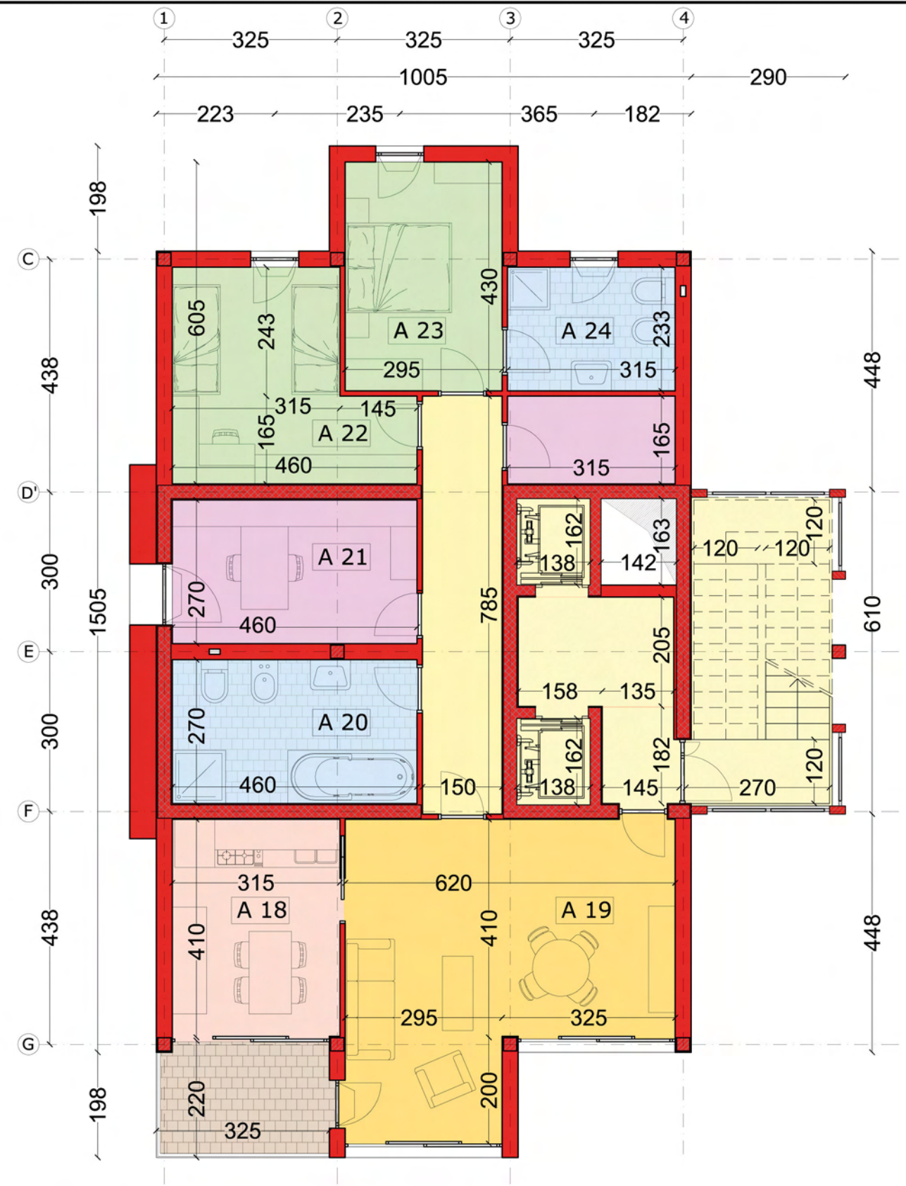
PIANTA TIPO "D"
