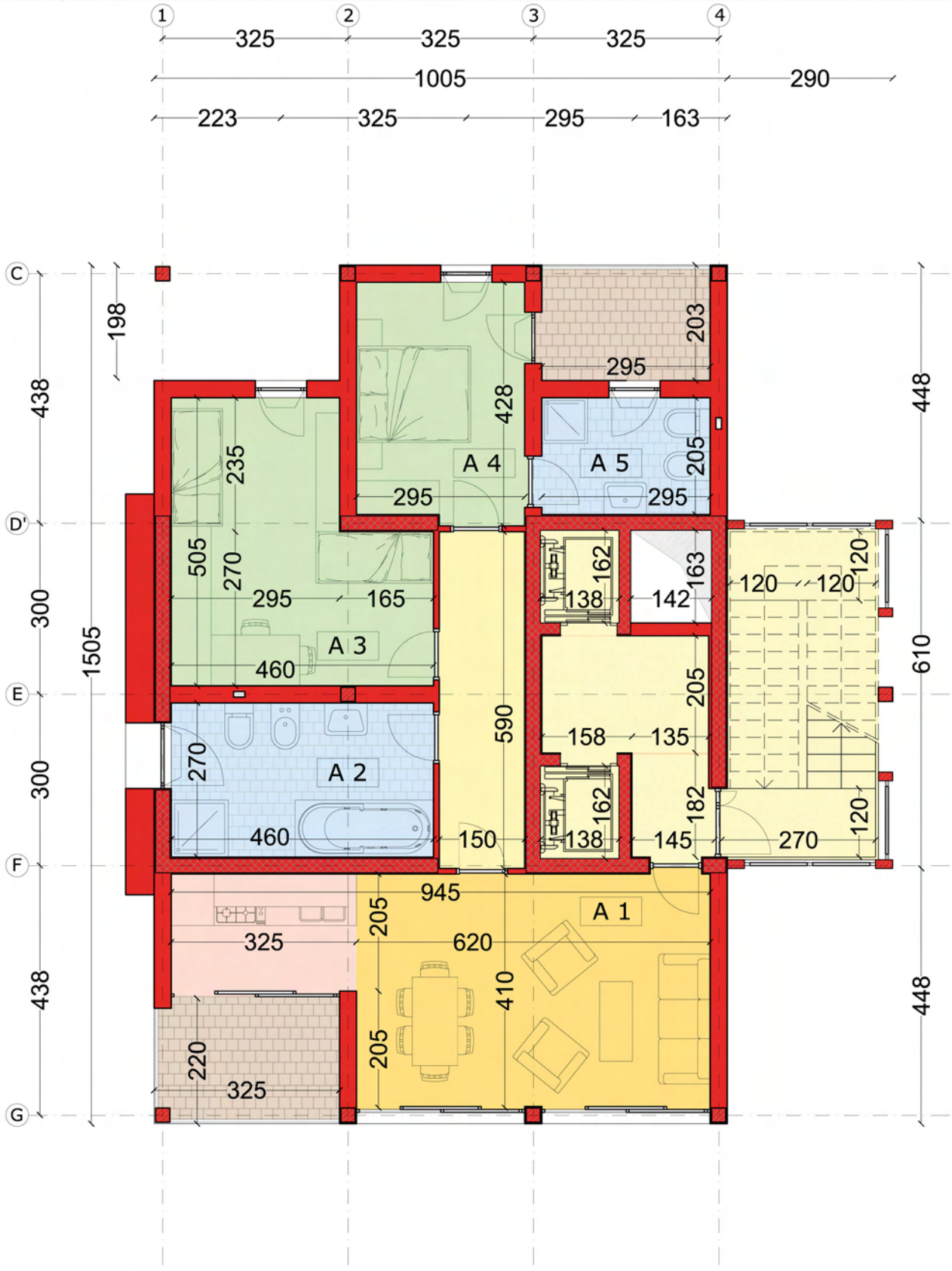
PIANTA TIPO "A"
