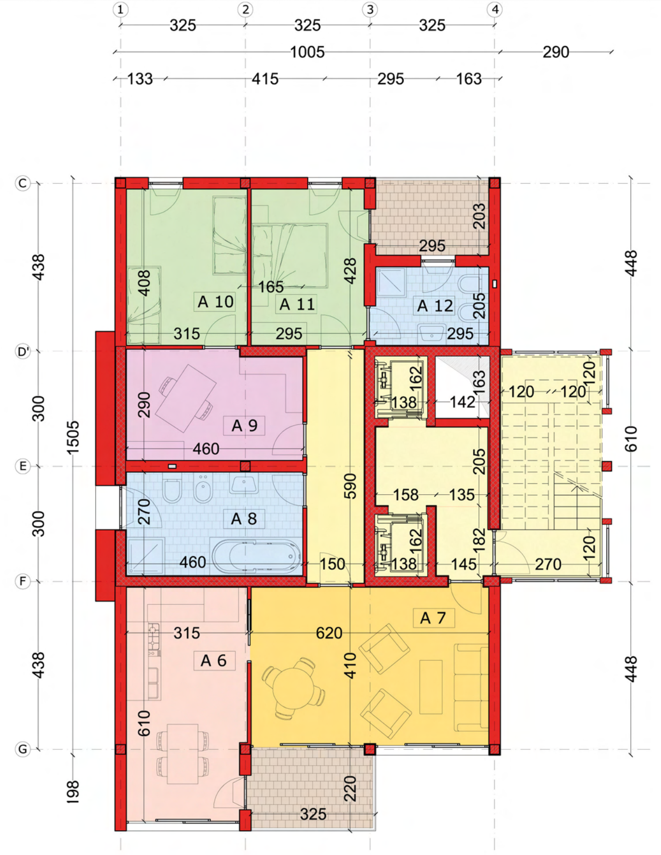
PIANTA TIPO "B"
