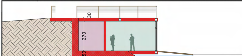
SEZIONE TIPO DEL NEGOZIO
