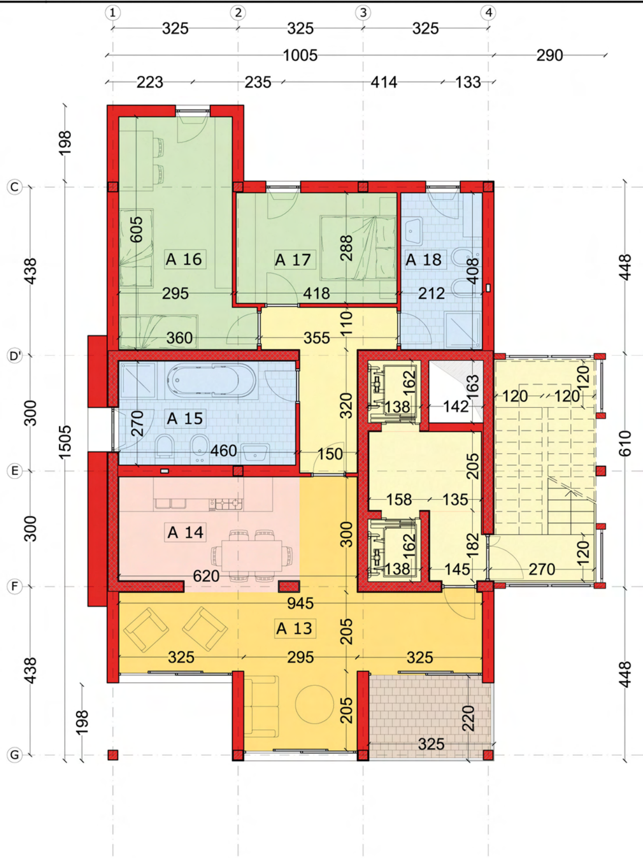
PIANTA TIPO "C"
