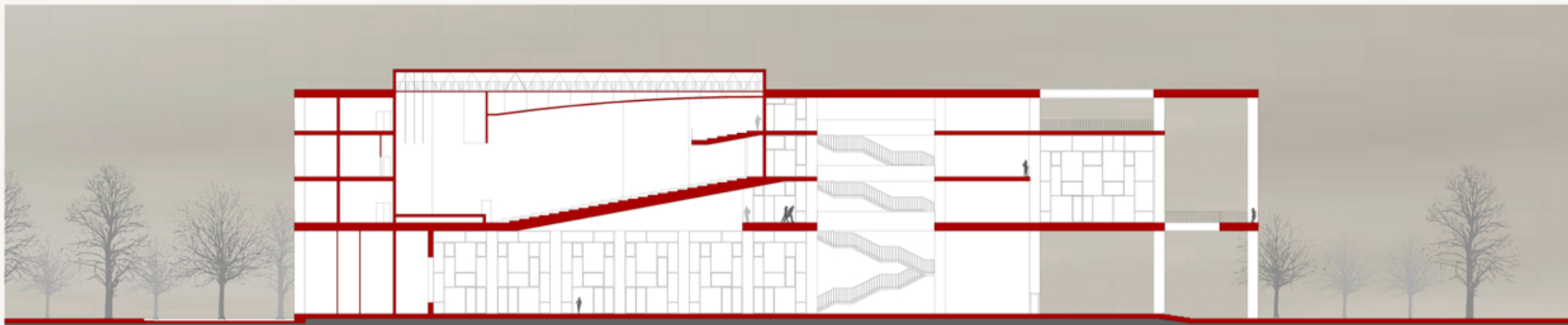
SEZIONE A-A
