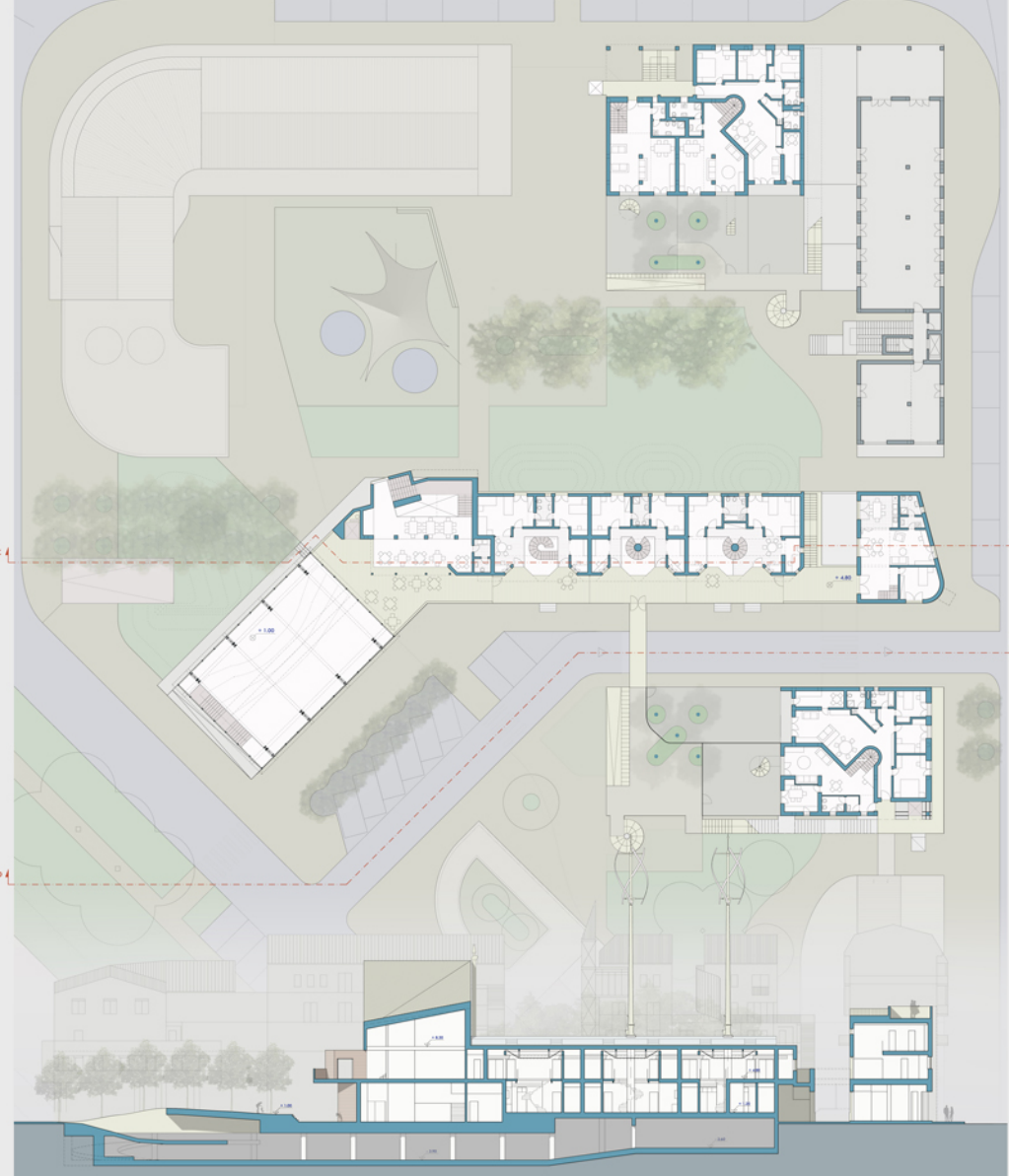
SEZIONE CC
