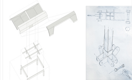
ORGANICO a DIMENSIONI, impostazione del nodo di connessione di un a rispetto la trama di copertura
