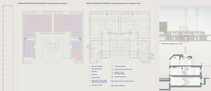
SCHEMA IMPIANTICO RISCALDAMENTO pannelli radianti a pavimento
