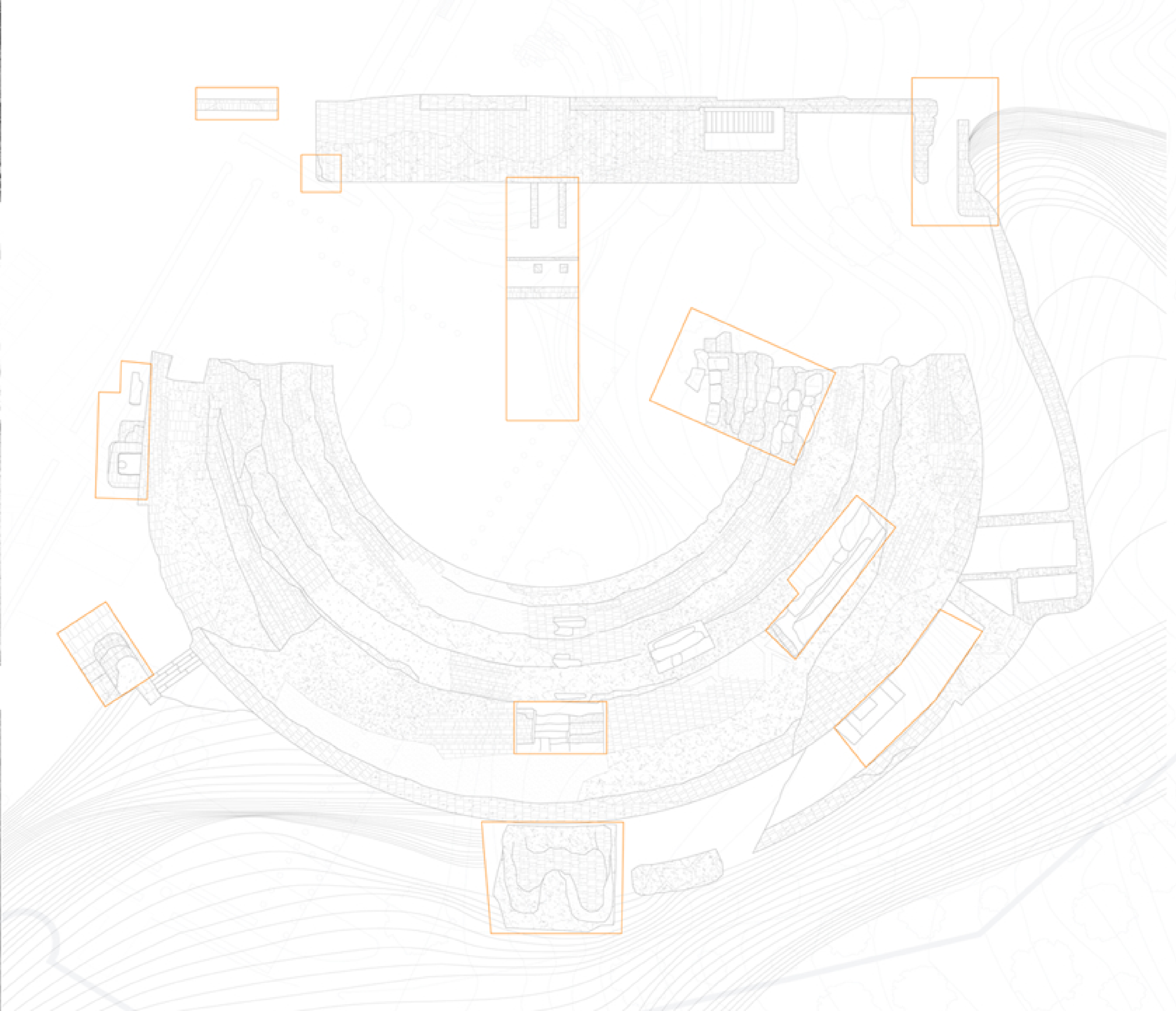
Pianta a quota +11.50 m con indicazione degli scavi
