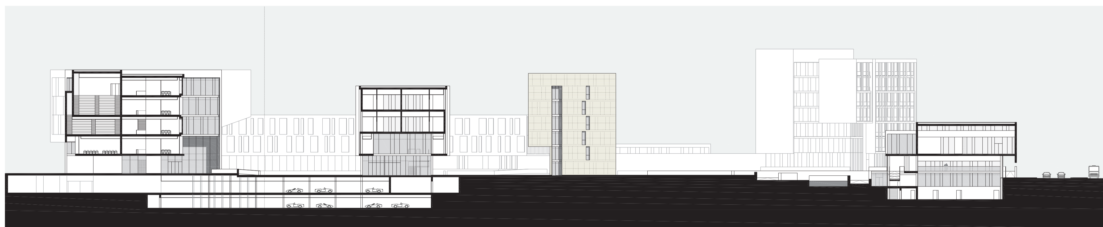
Sezione FF _scala 1 500
