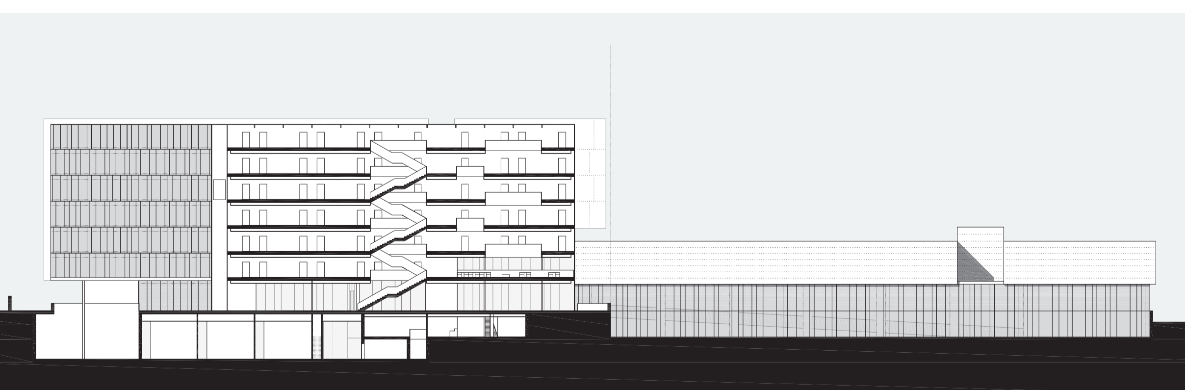
Sezione SS _scala 1 500
