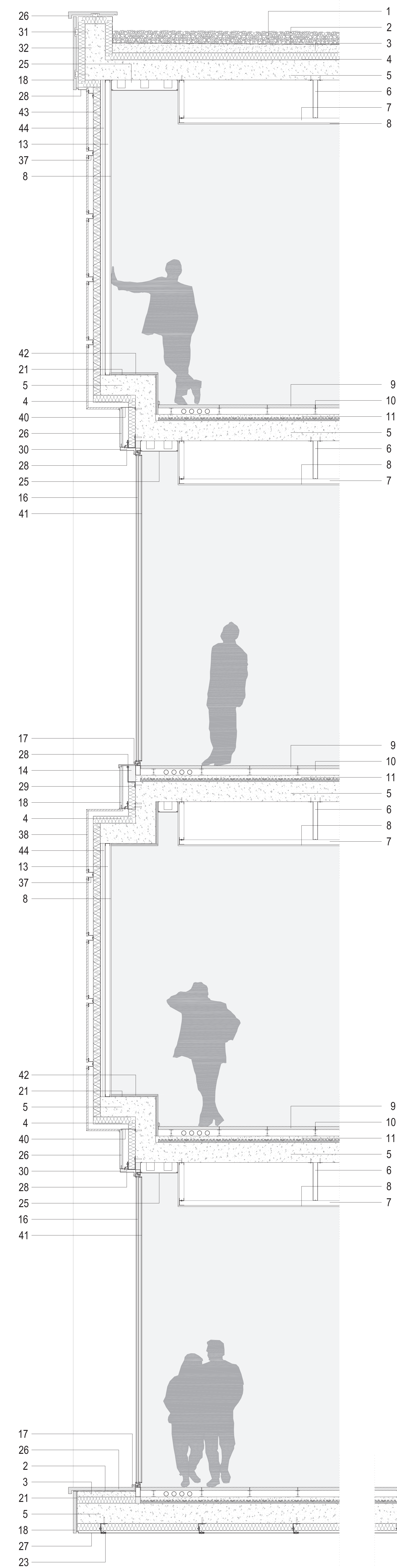
Comparto didattico: dettaglio della facciata sud _scala 1 20
