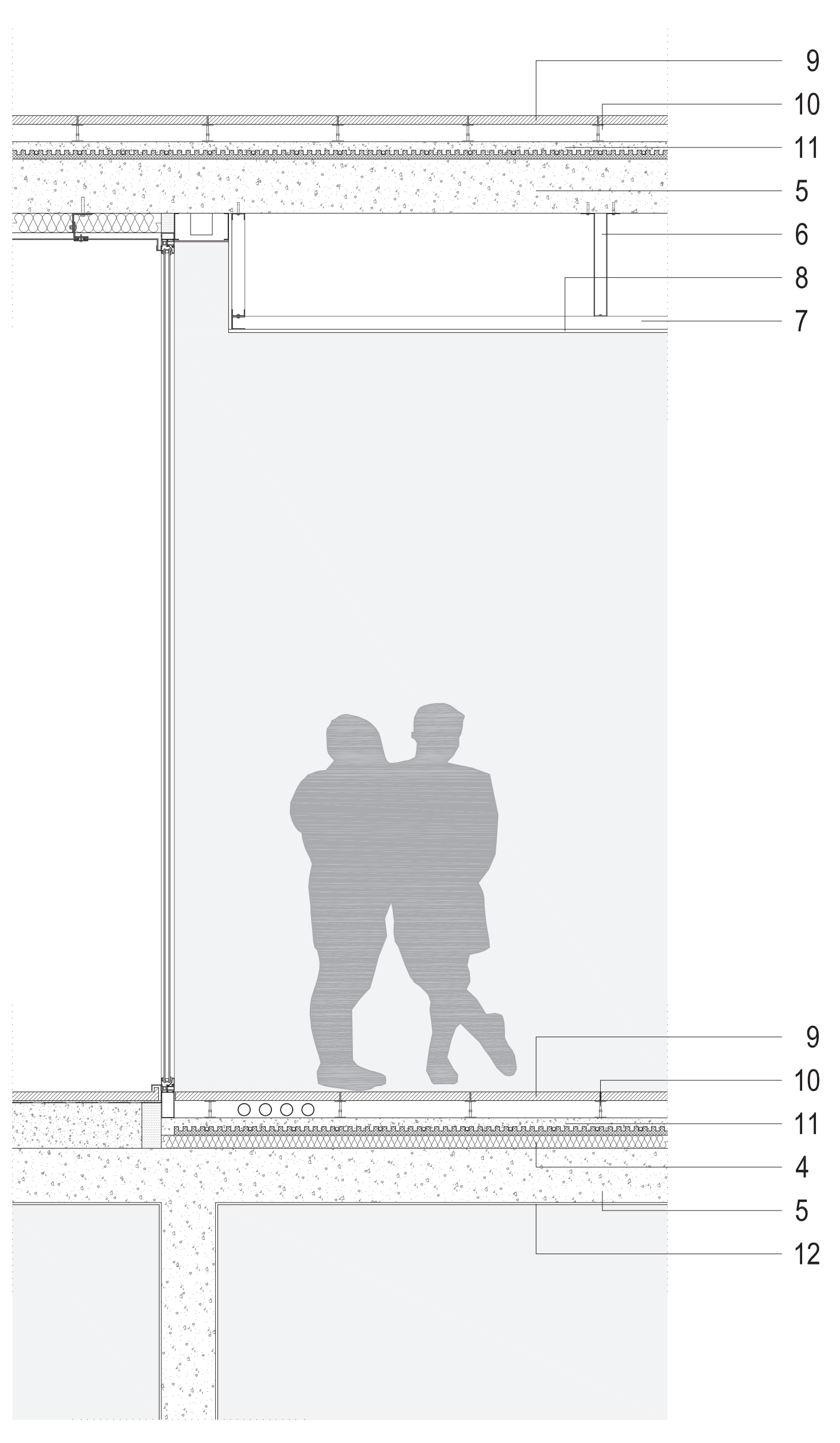
Sezione prospettica del comparto didattico
