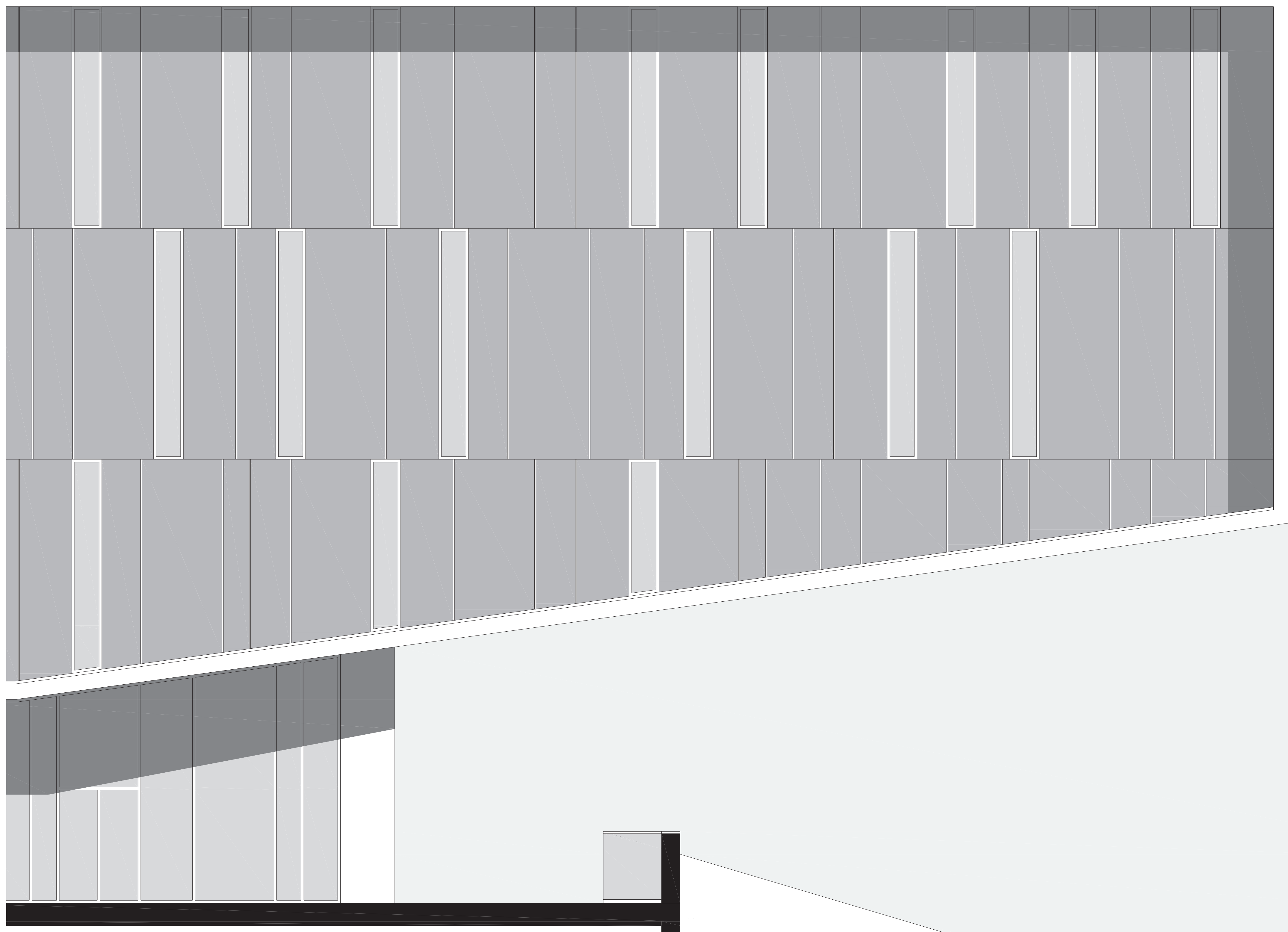
Porzione significativa del prospetto sud _scala 1 50
