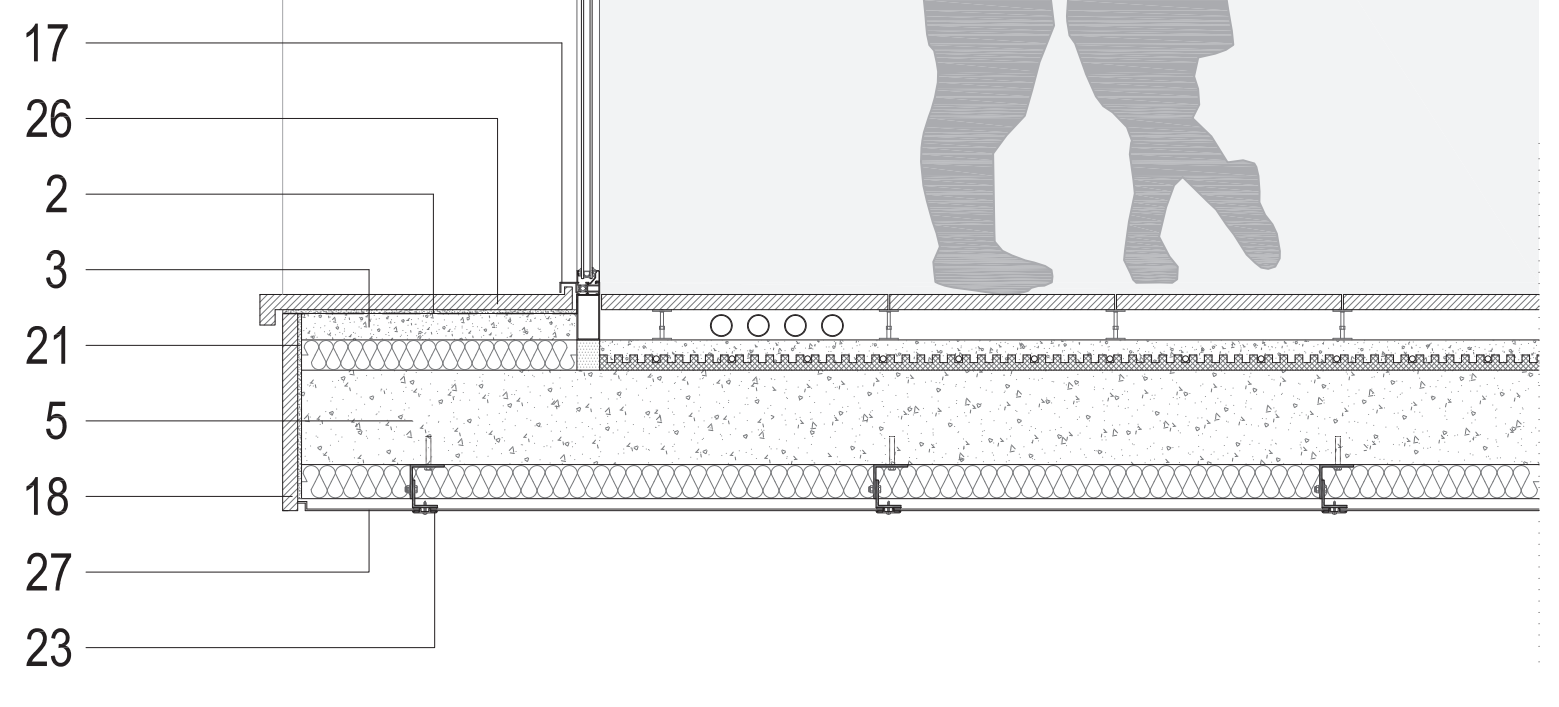
Student Center: dettaglio della facciata sud _scala 1 20
