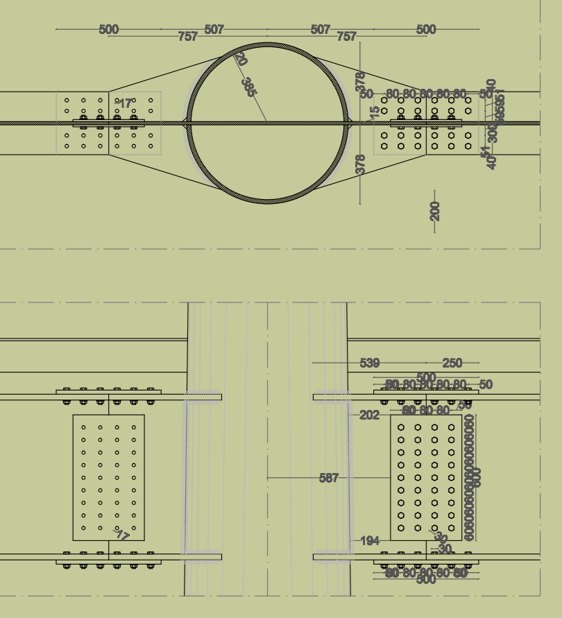
sezione CC collegamento tra colonna tubolare e trave principale scala 1:25
