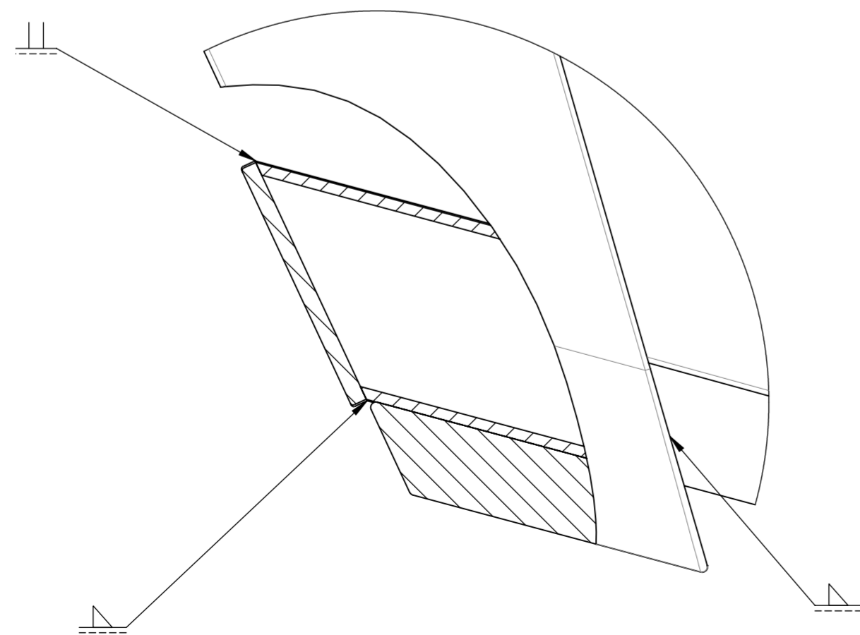
DETTAGLIO A SCALA 1 : 1
