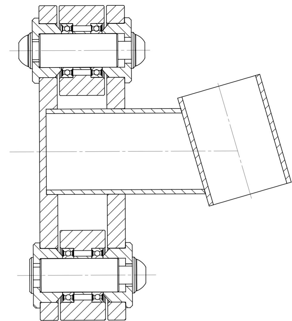
SEZIONE A-A SCALA 1 : 1
