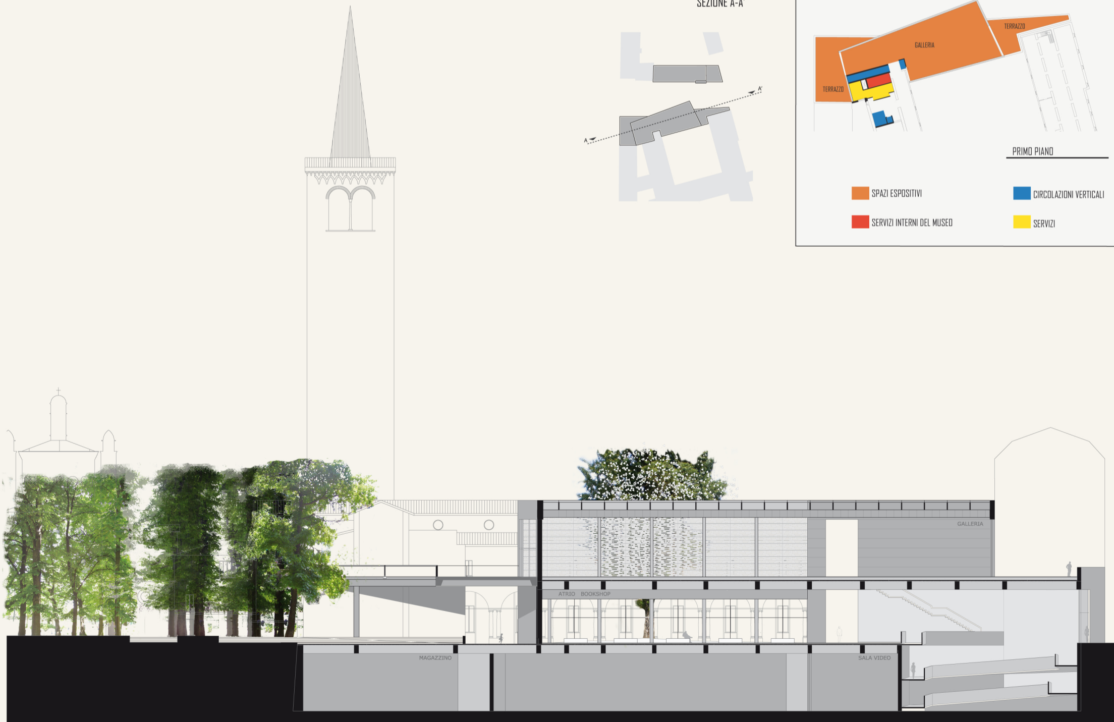
SEZIONE A-A'
