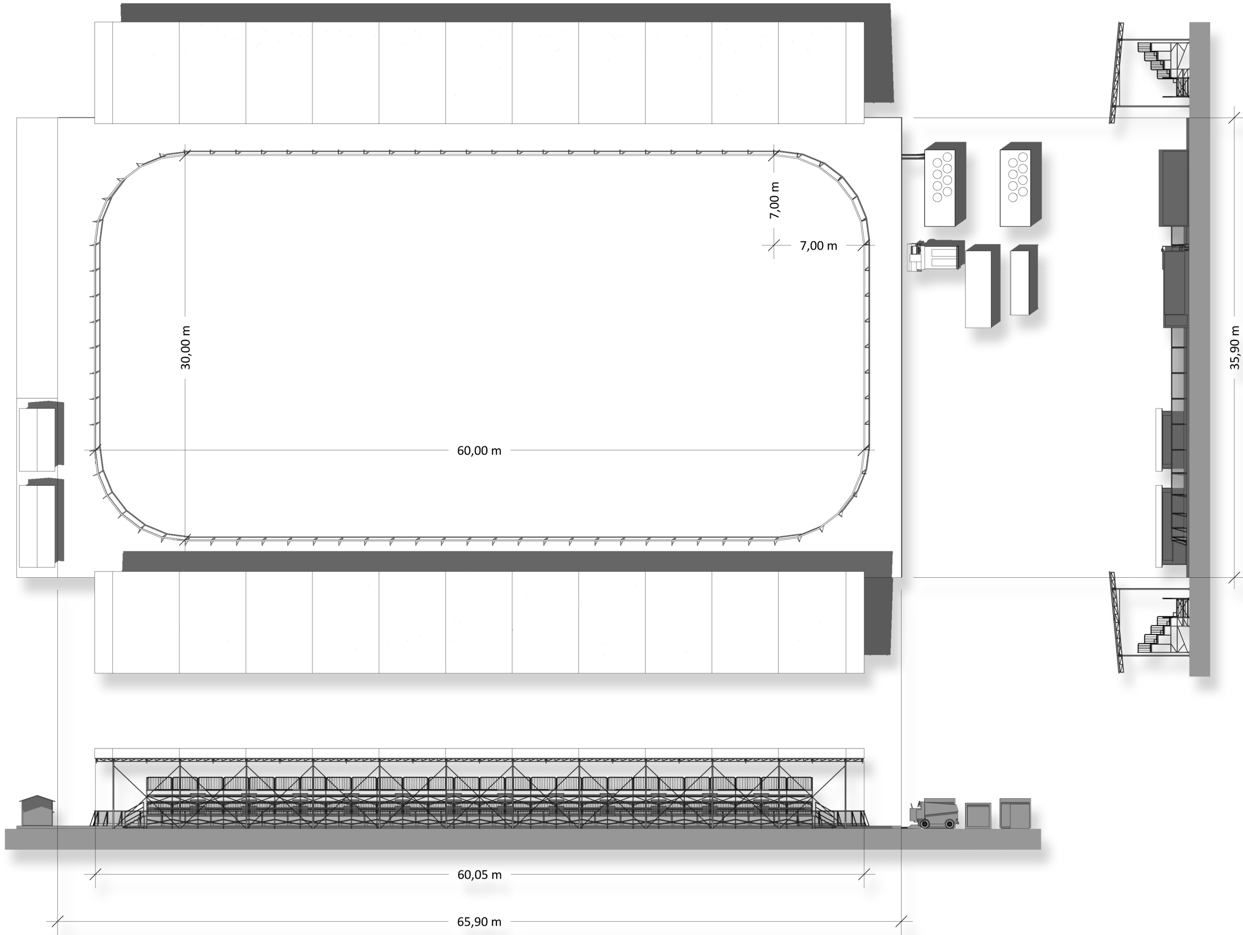
PROSPETTO LATERALE
