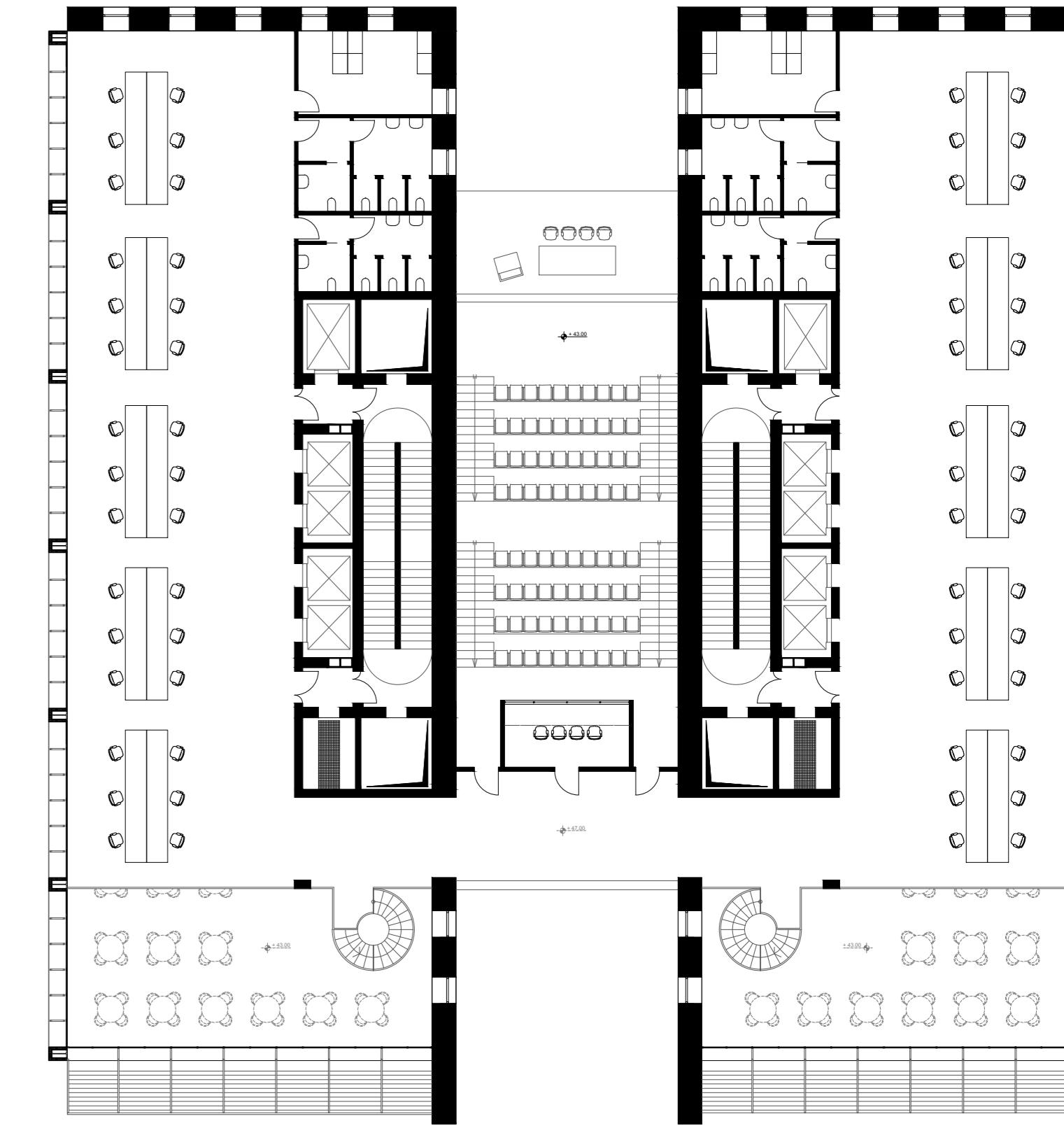
PIANI 11-20
