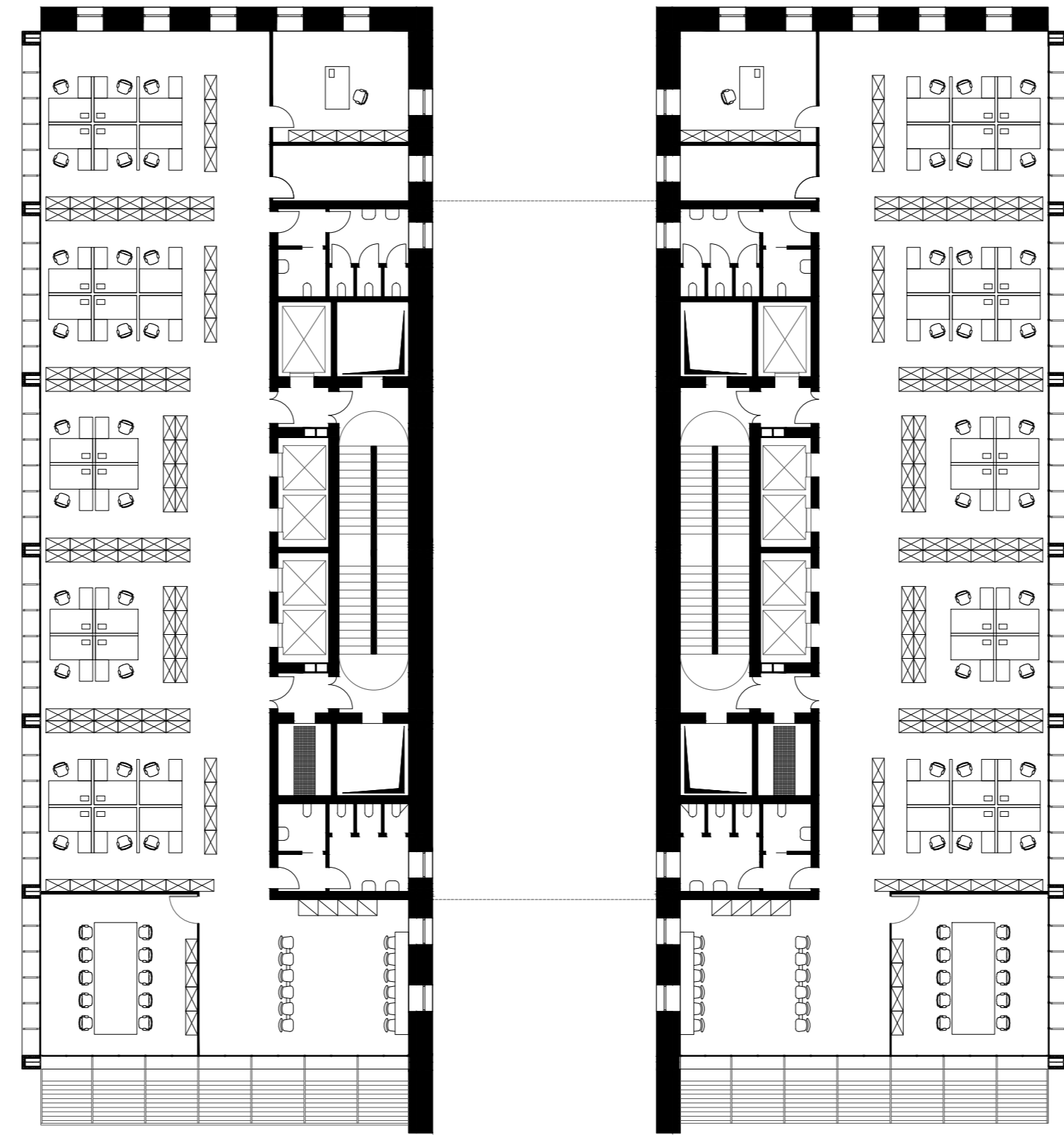
PIANO TIPO
