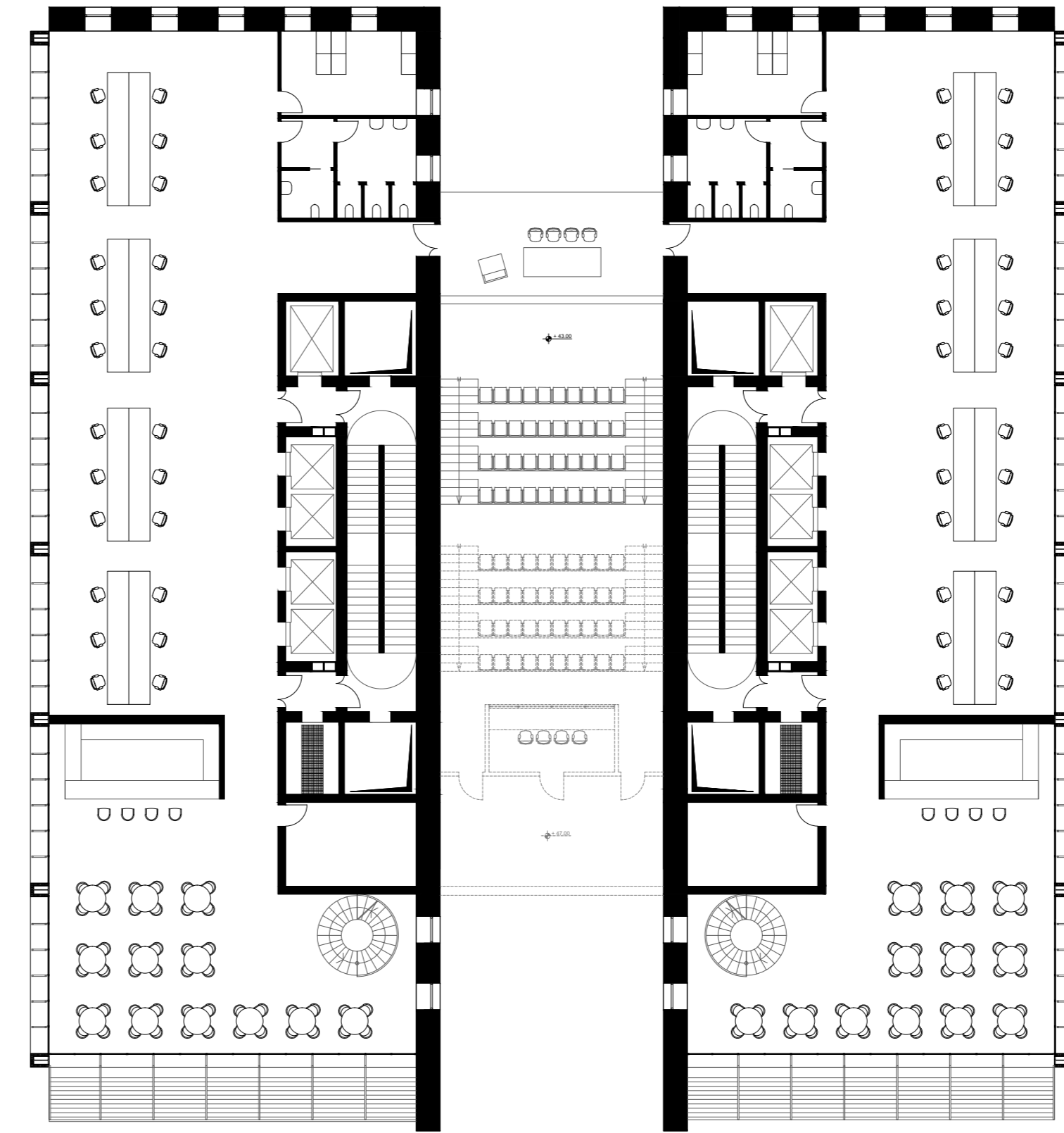
PIANI 10-19
