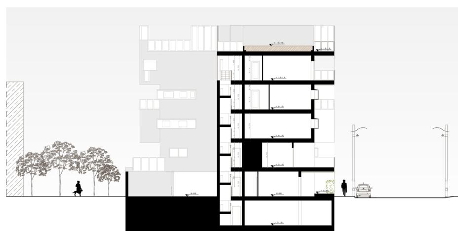
SEZIONE B_B'
