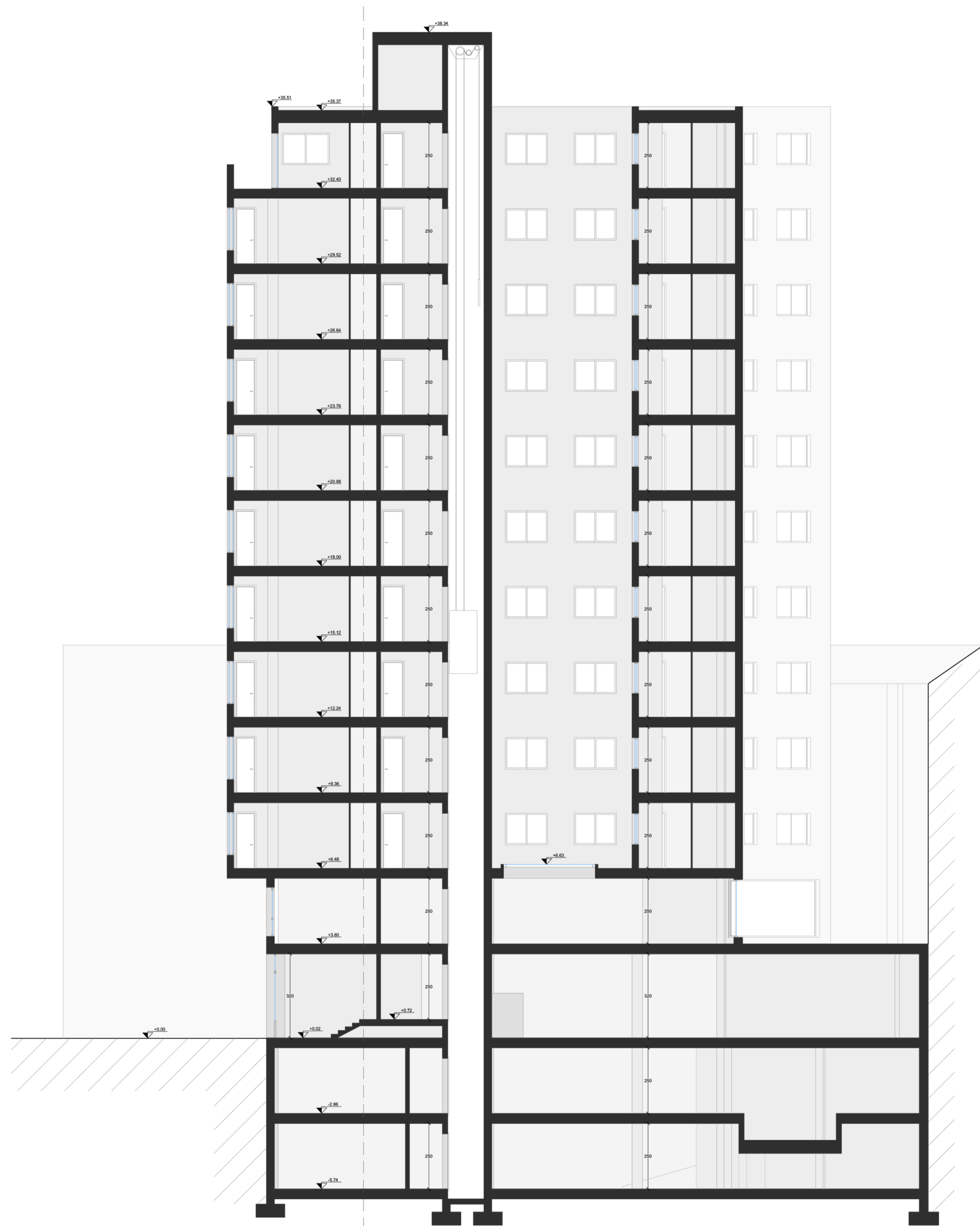
SEZIONE A-A'
