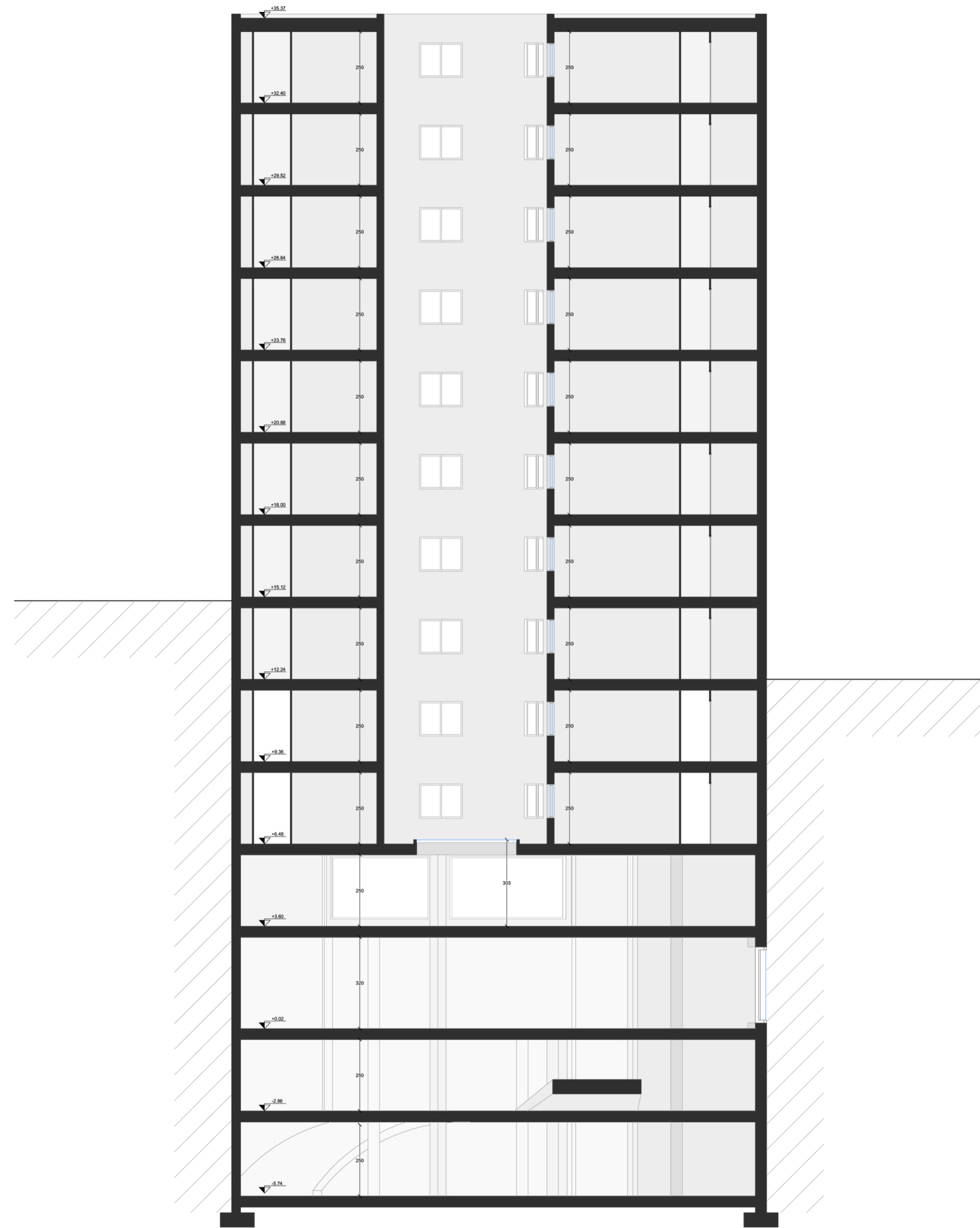
SEZIONE B-B'
