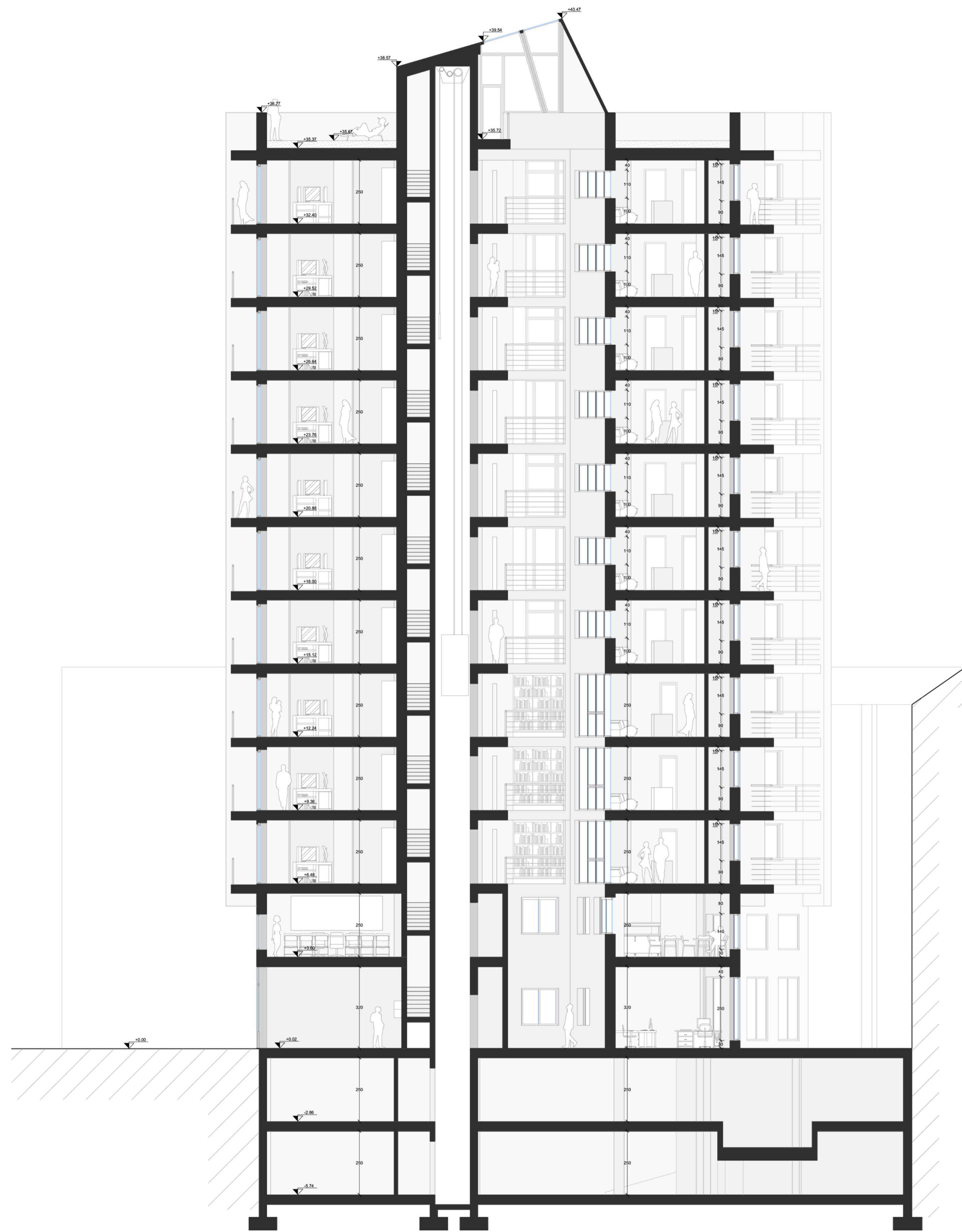
SEZIONE A-A'
