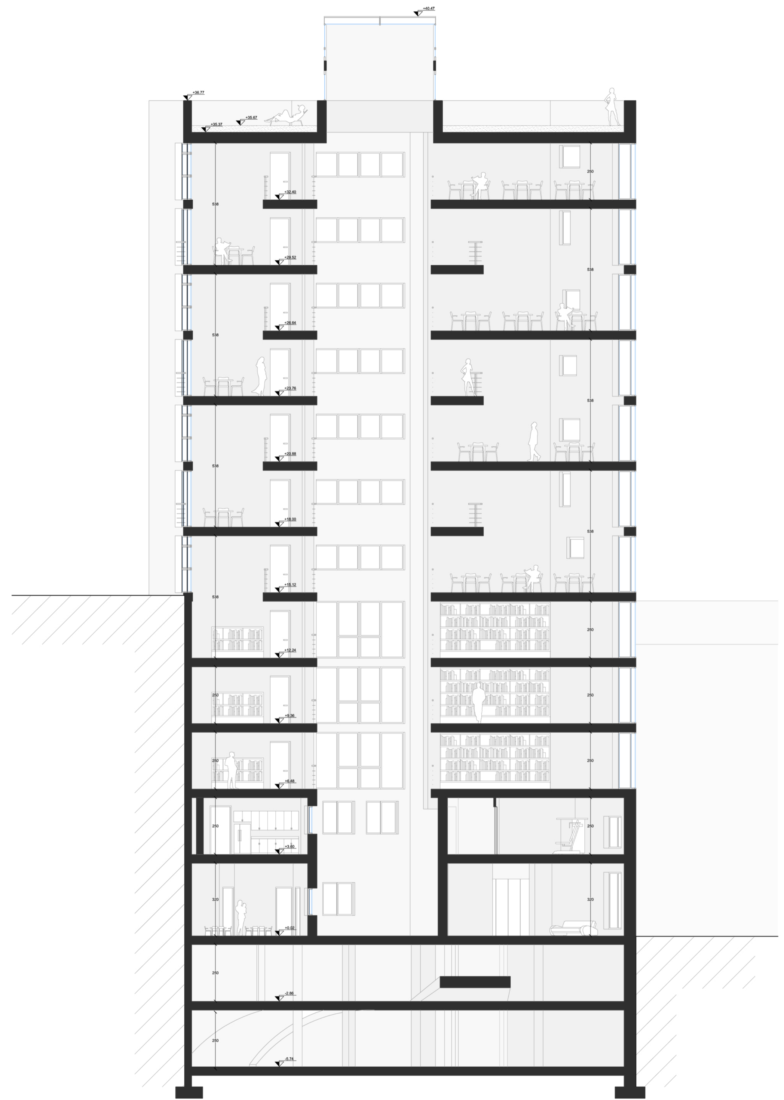
SEZIONE B-B'
