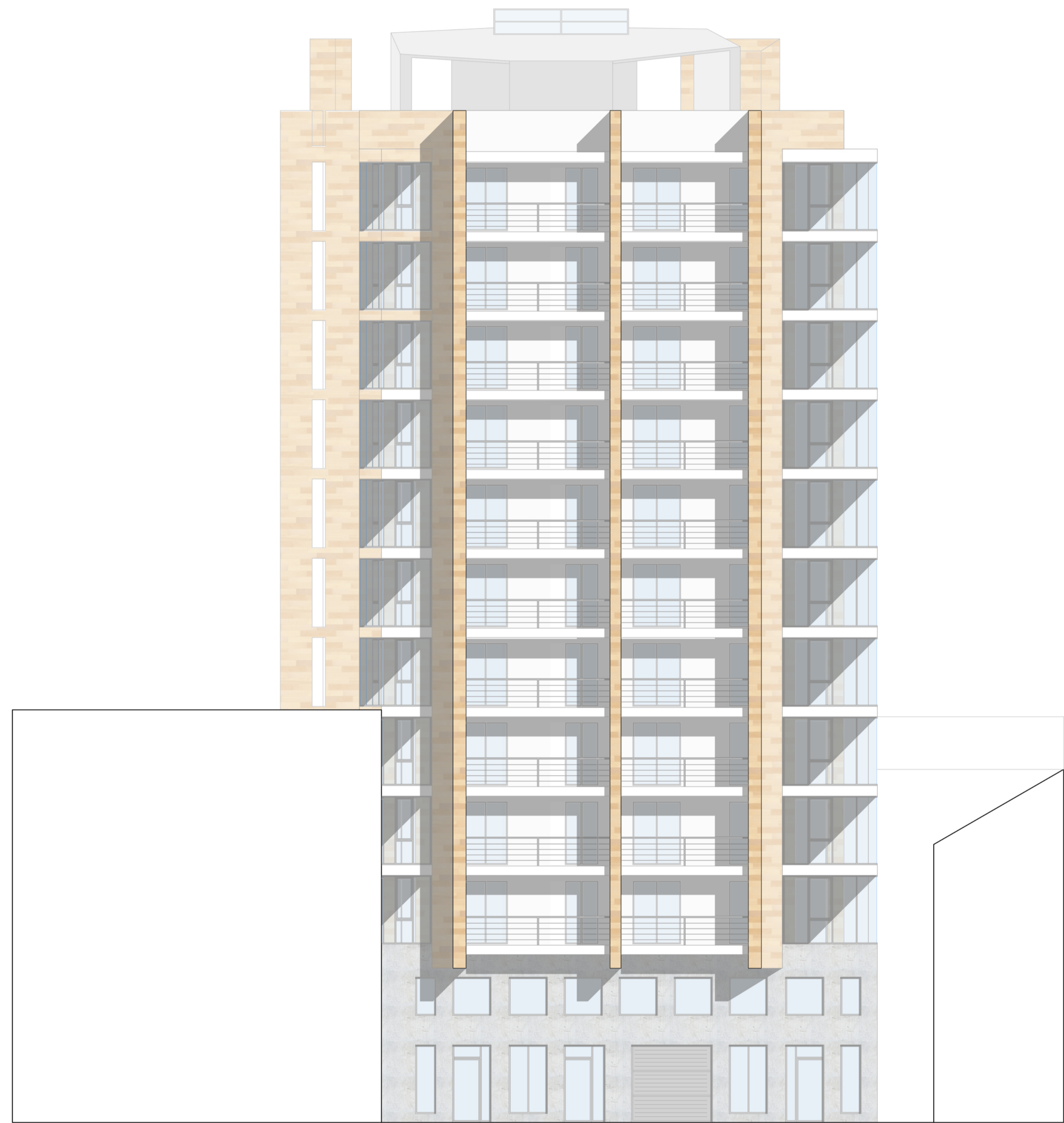
PROSPETTO SUD
