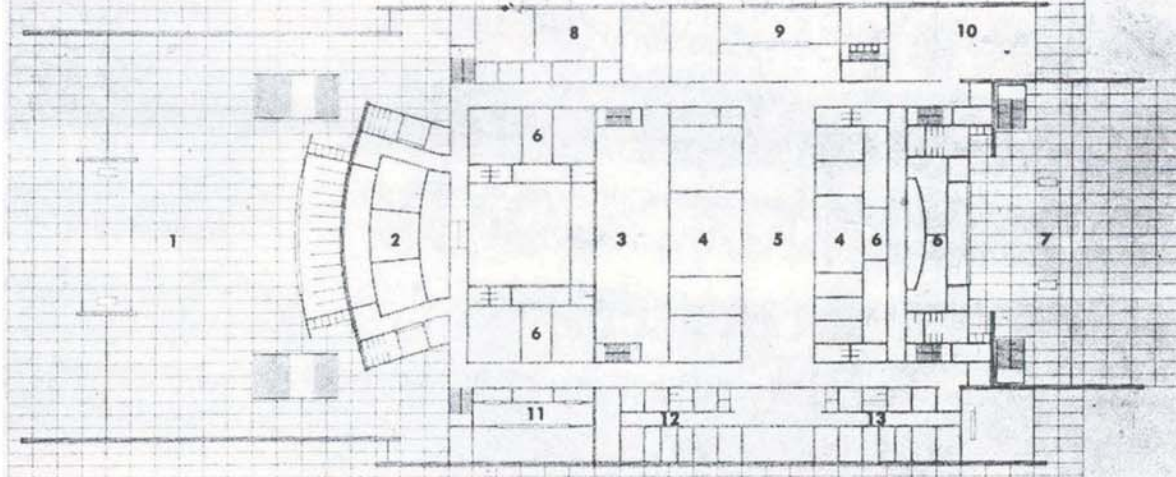
TEATRO DI MANNHEIM
