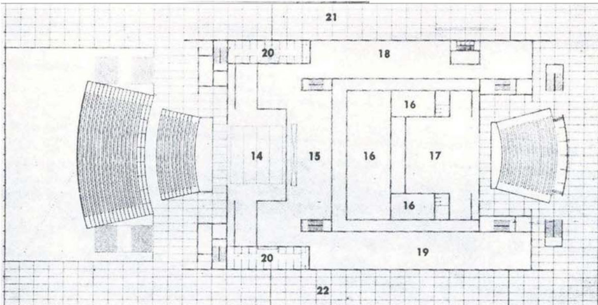
TEATRO DI MANNHEIM
