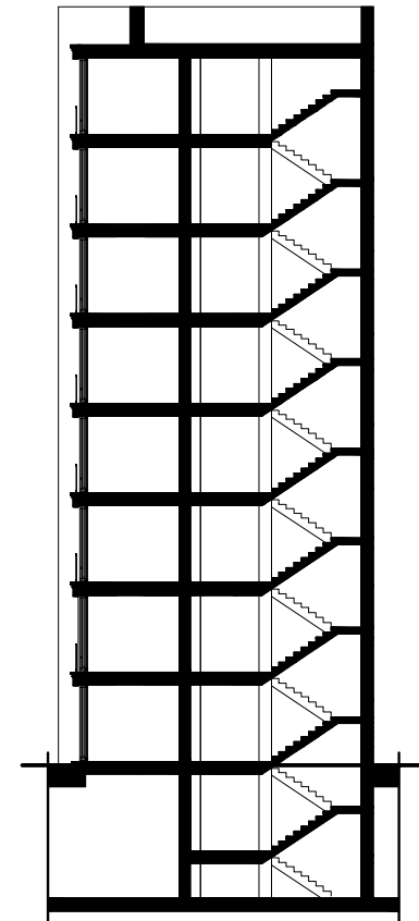
SEZIONE TRASVERSALE SUL SOGGIORNO
