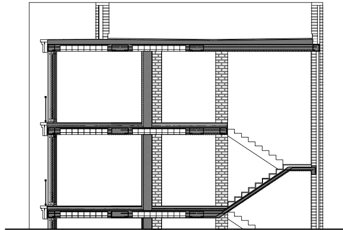
SEZIONE COSTRUTTIVA PER IL SOGGIORNO
