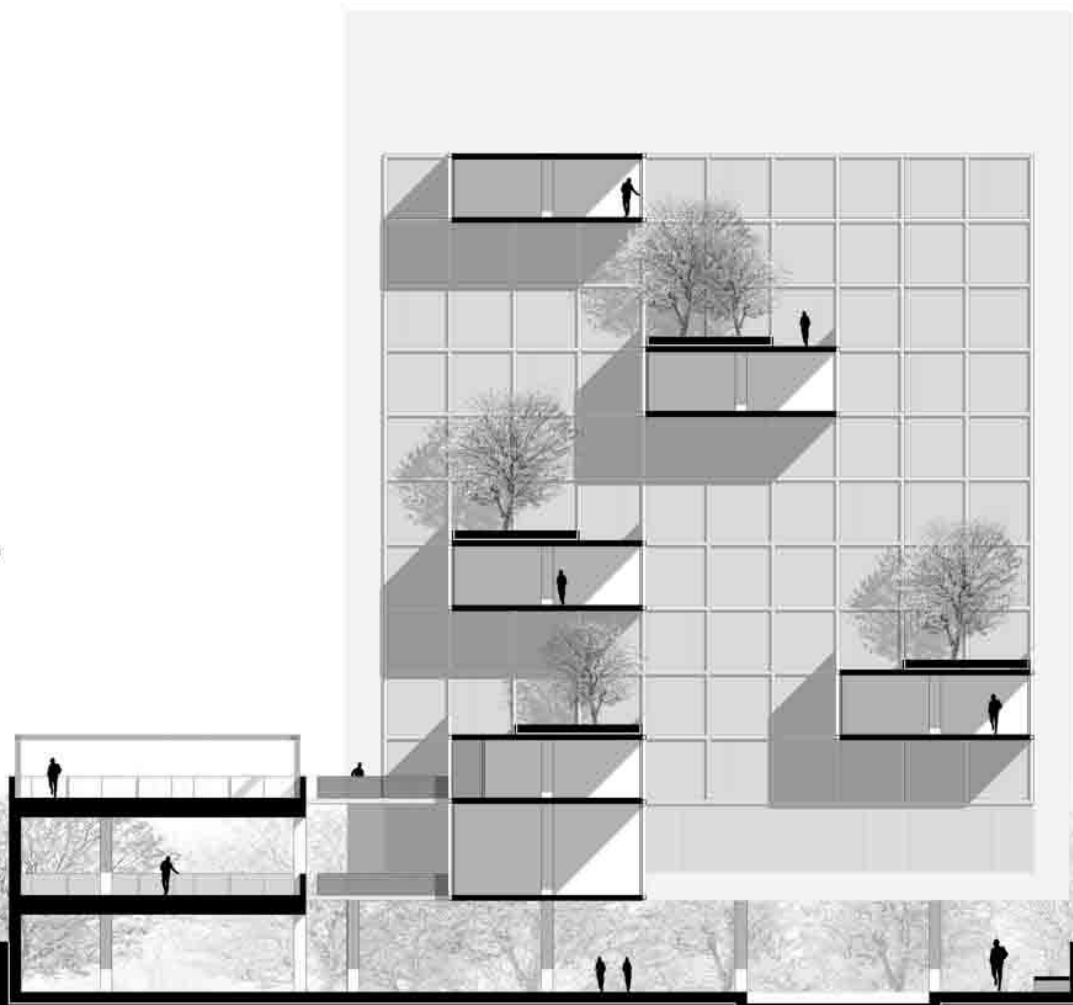
Sezione trasversale 0-0 scala 1:200
