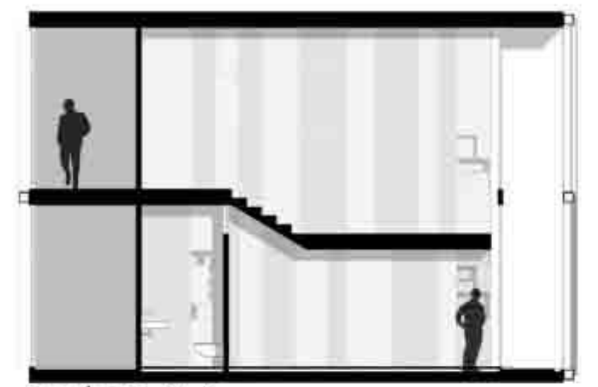
Sezione A-A scala 1:100
