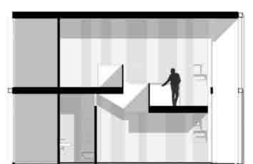
Sezione B-B scala 1:100
