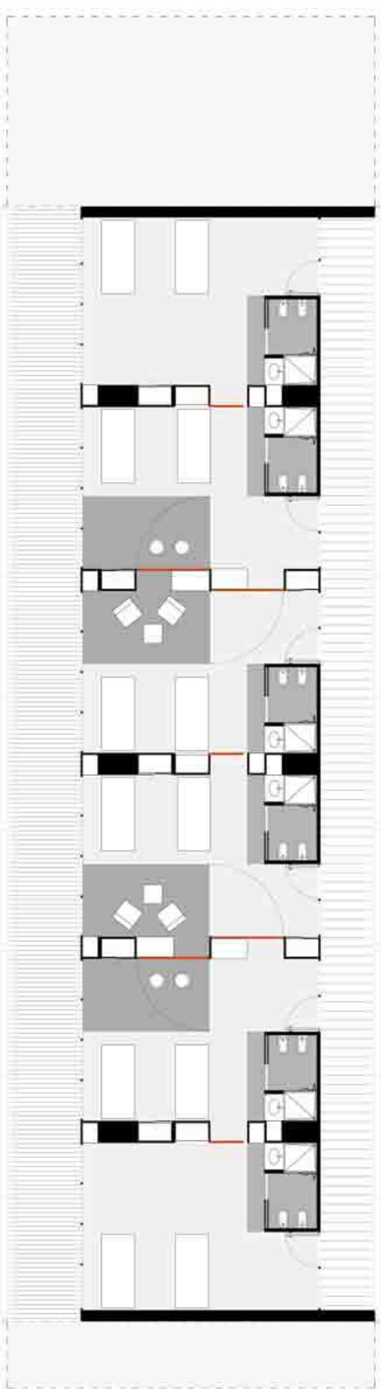
Volume Sud Pianta tipo Combinazione "CHIUSA" [n°1] scala 1:100
