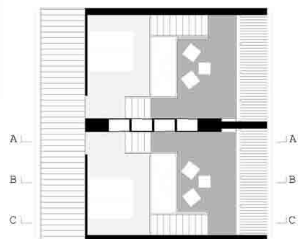
Pianta secondo livello scala 1:100
