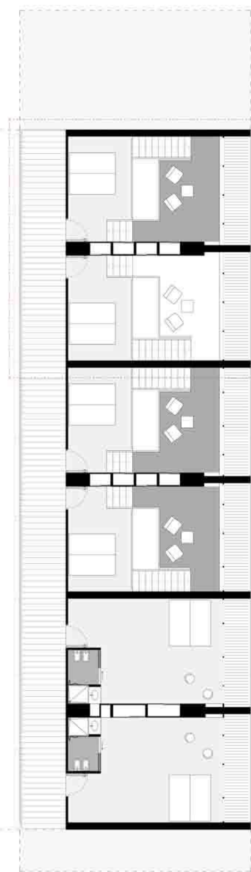
Volume Nord Pianta tipo DUPLEX scala 1:100
