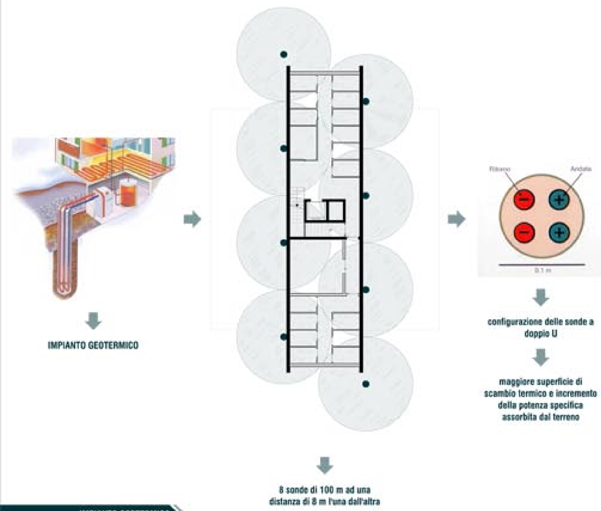
IMPIANTO GEOTERMICO
