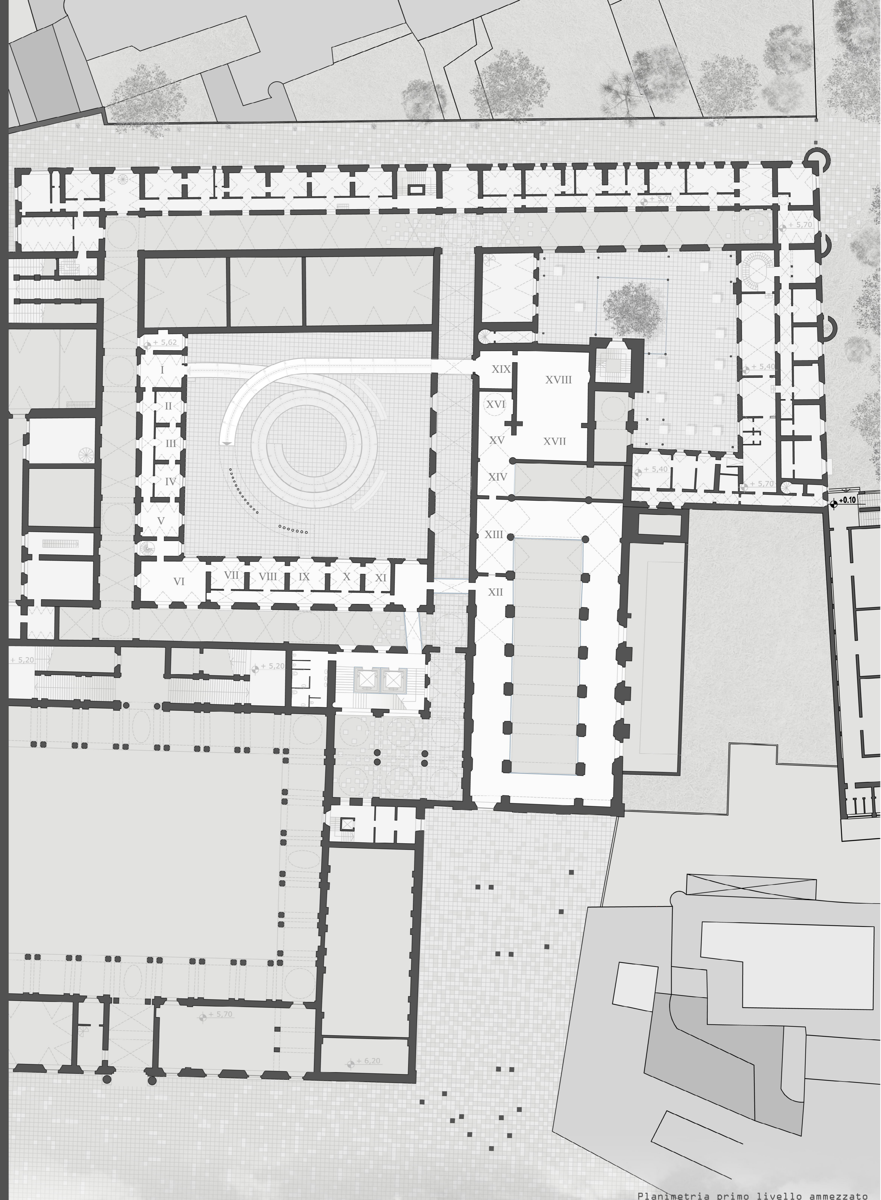
Planimetria primo livello ammezzato Scala 1:300
