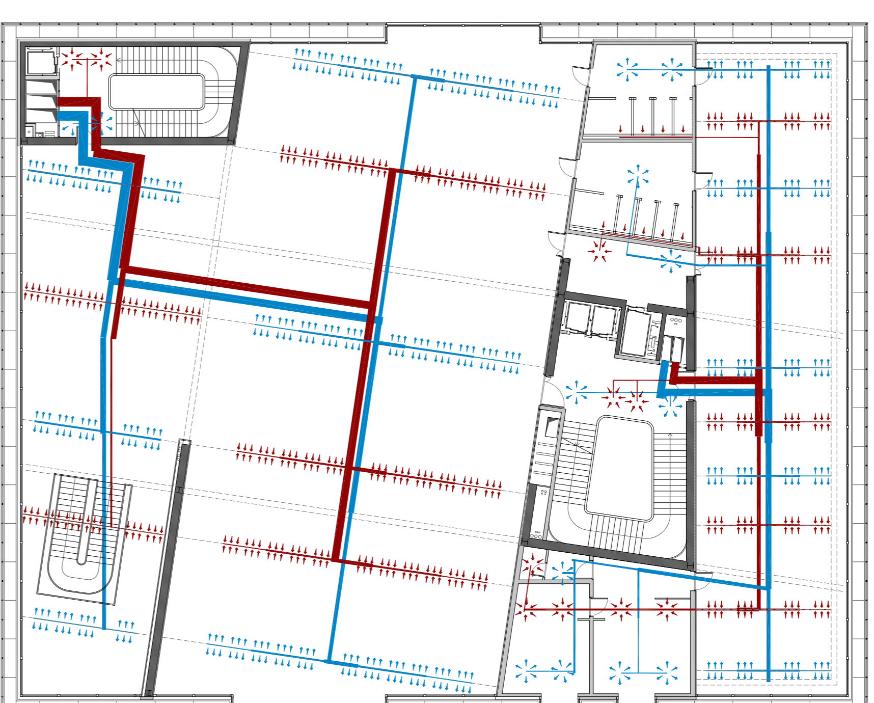
Piano primo
