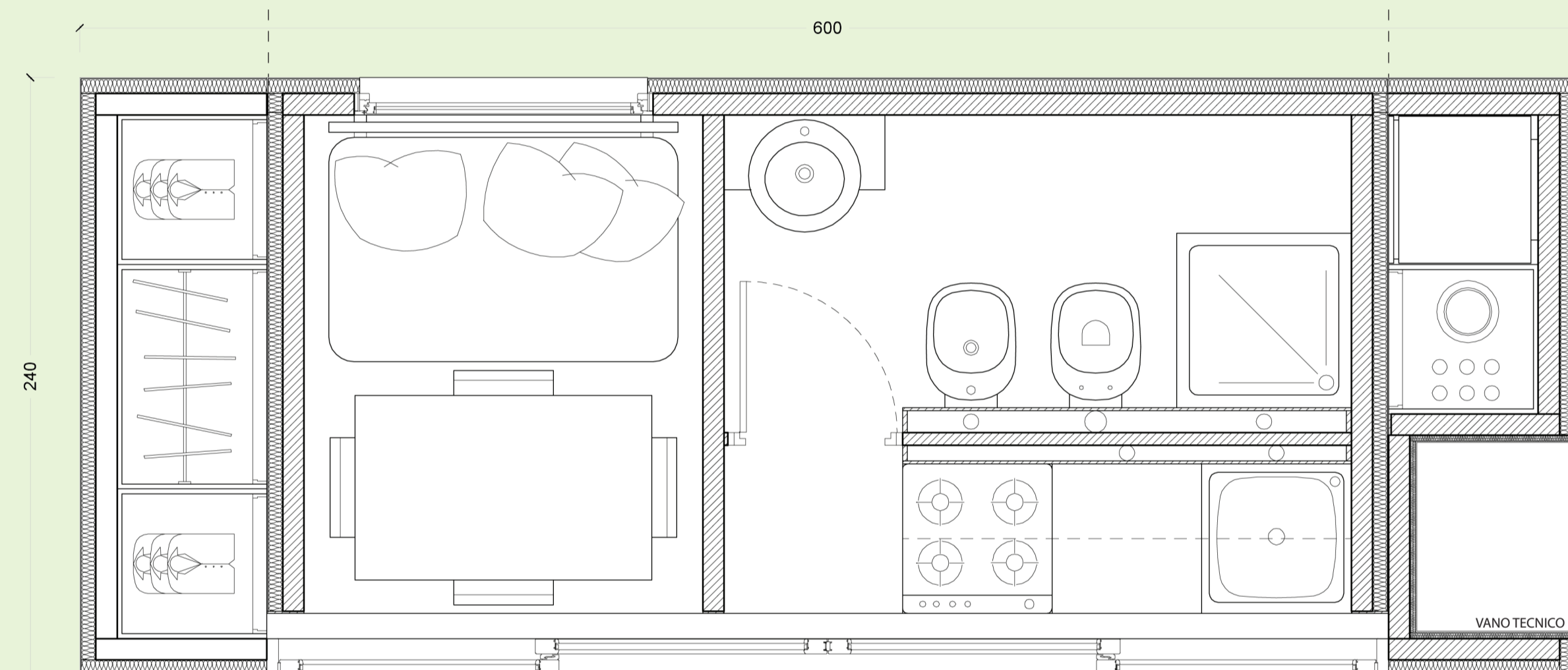
PIANTA MODULO CHIUSO PER TRASPORTO 11,4 mq
