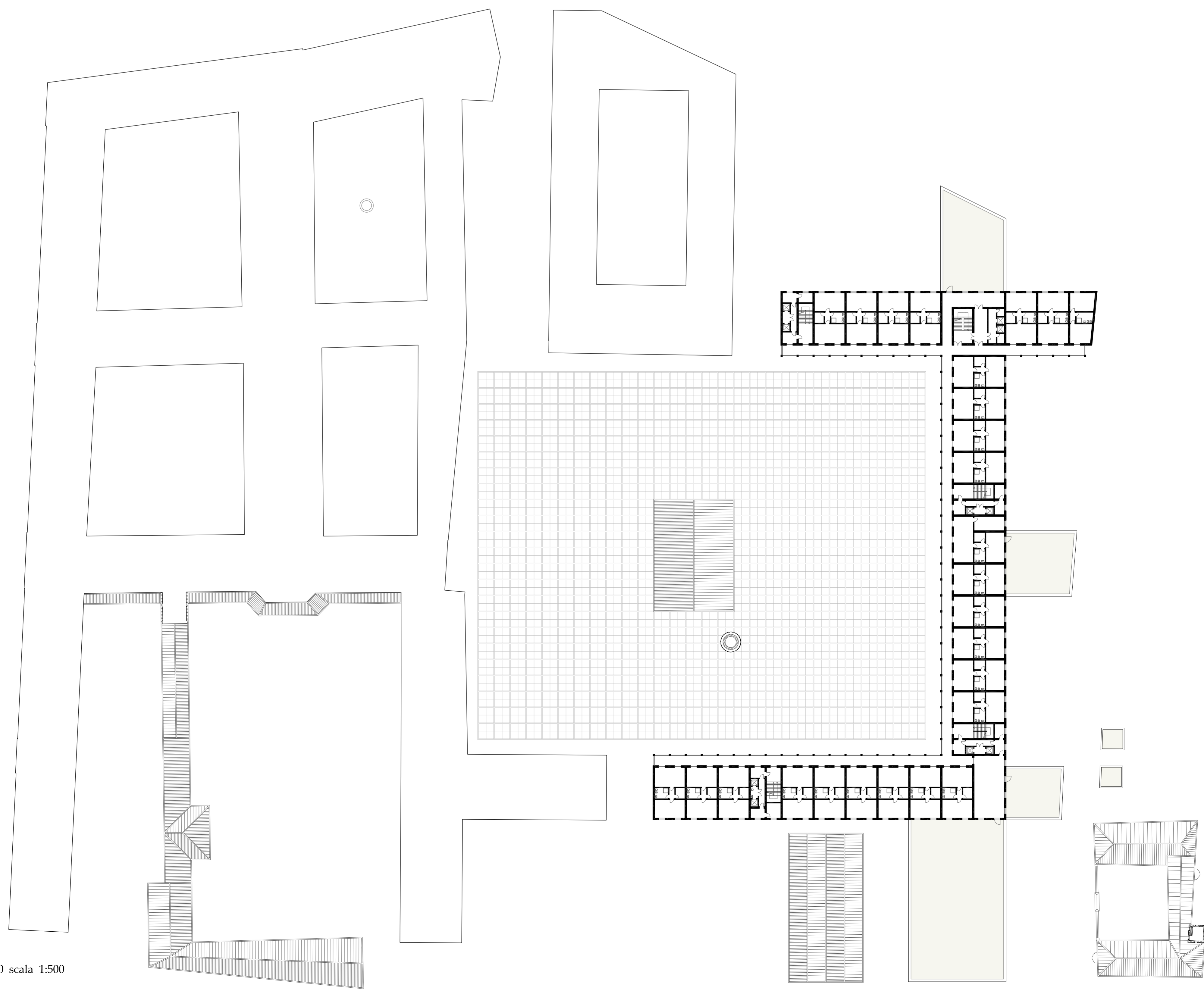
pianta quota +3,80 scala 1:500
